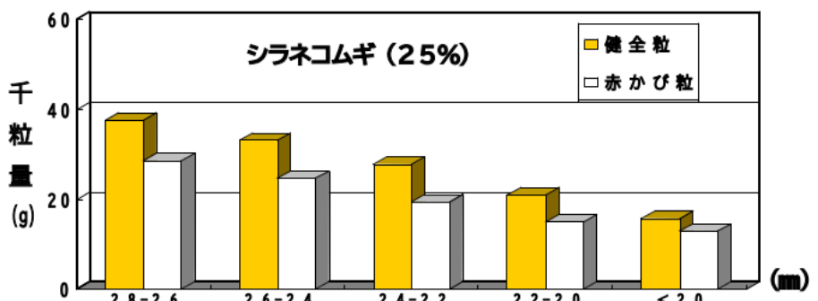
図1 健全粒および赤かび粒の粒厚別千粒重(古川農試 平17) 注( )内の数字は出穂約40日後における発病率
