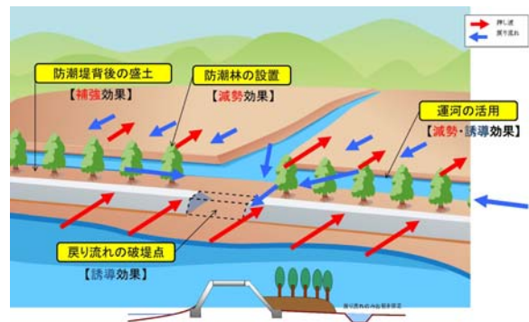
図-5 海岸保全施設の「粘り強い」構造のイメージ
