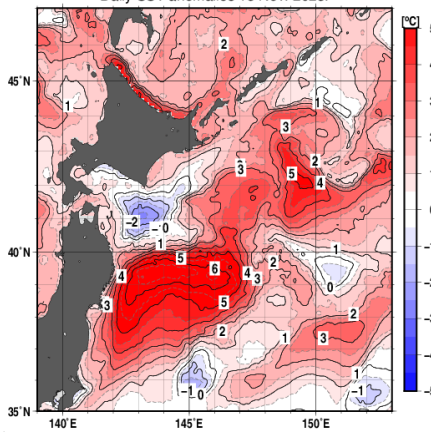
Daily SST anomalies 15 Nov. 2023.
