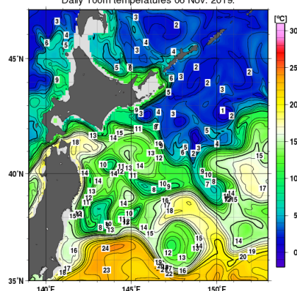
100 m深水温
