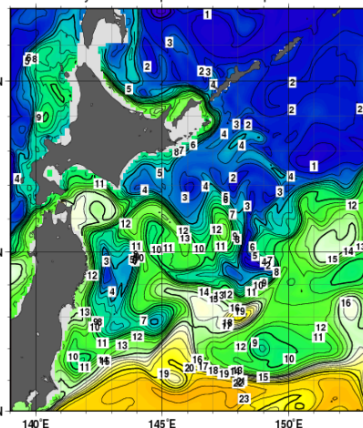
100 m深水温
