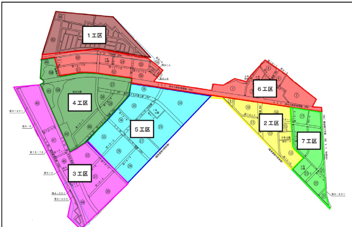
出来形確認測量実施状況図
