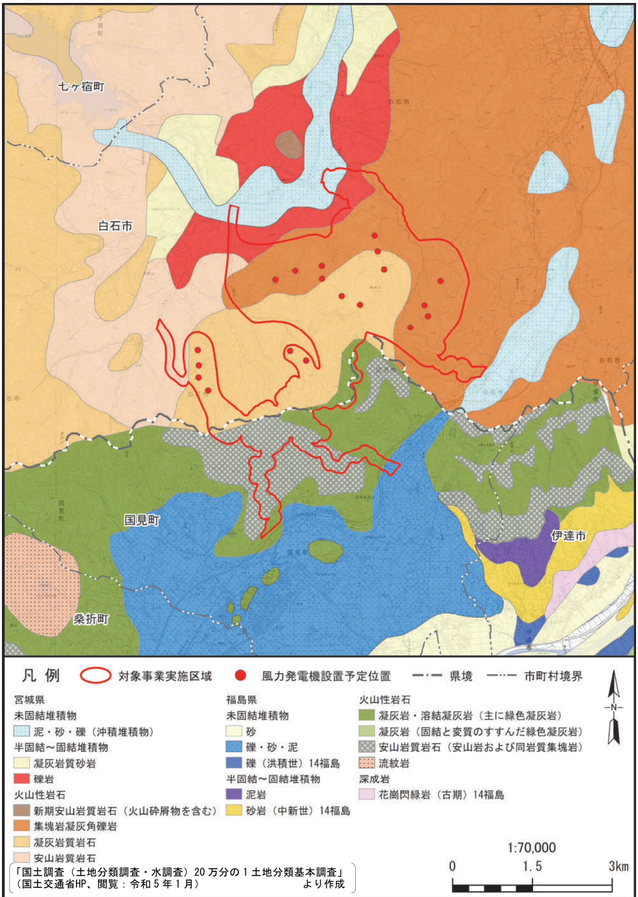
第 3.1.4-2 図 表層地質
