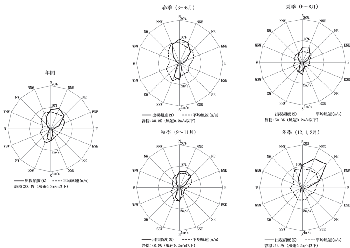
第 3.1.1-3 図 茂庭地域気象観測所の風配図（令和 4 年）
