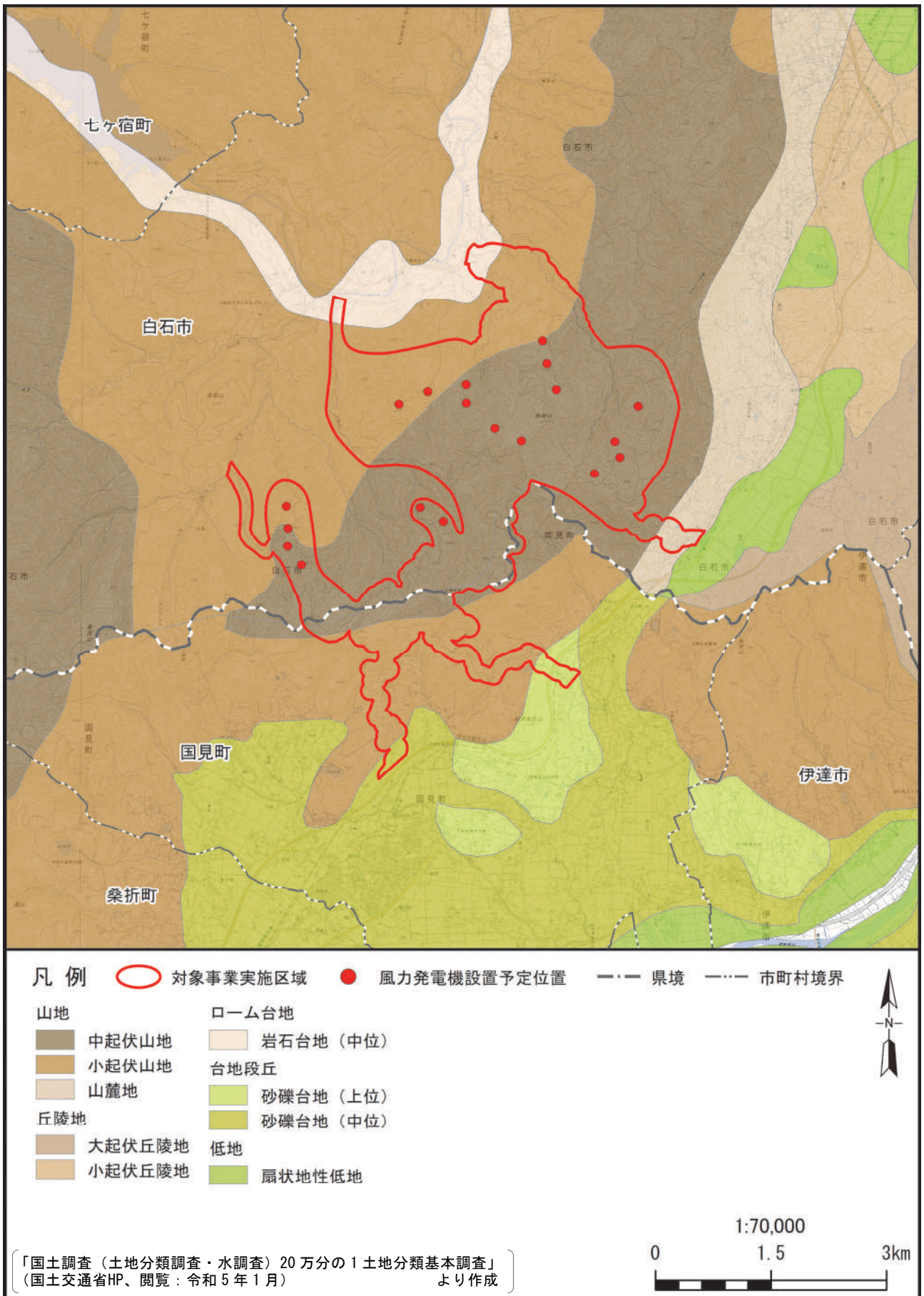
第 3.1.4-1 図 地形分類図
