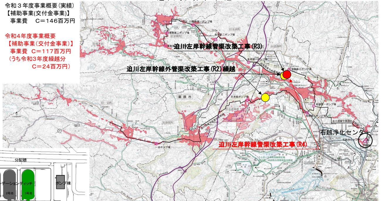
石越浄化センター一般平面図
