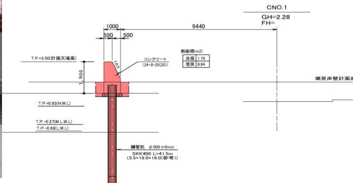
潮見地区防潮堤 標準断面図 S=1:100
