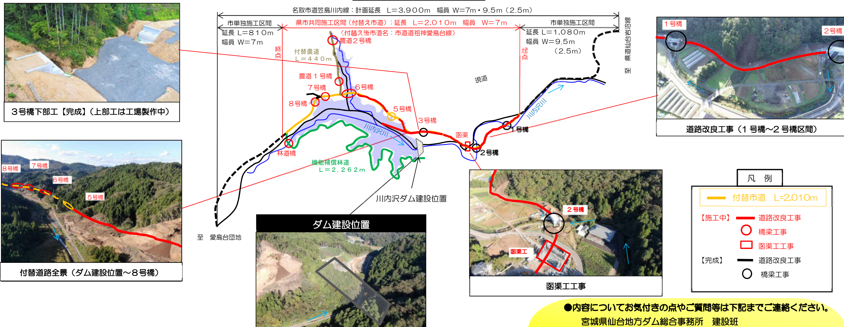
川内沢ダム建設事業全体平面図
