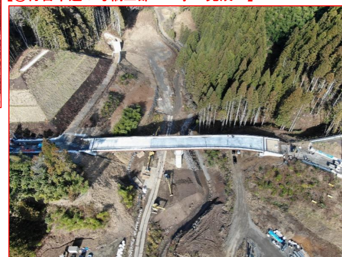
【②付替市道6号橋上部工工事 完成！】
