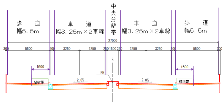
【標準横断図】
