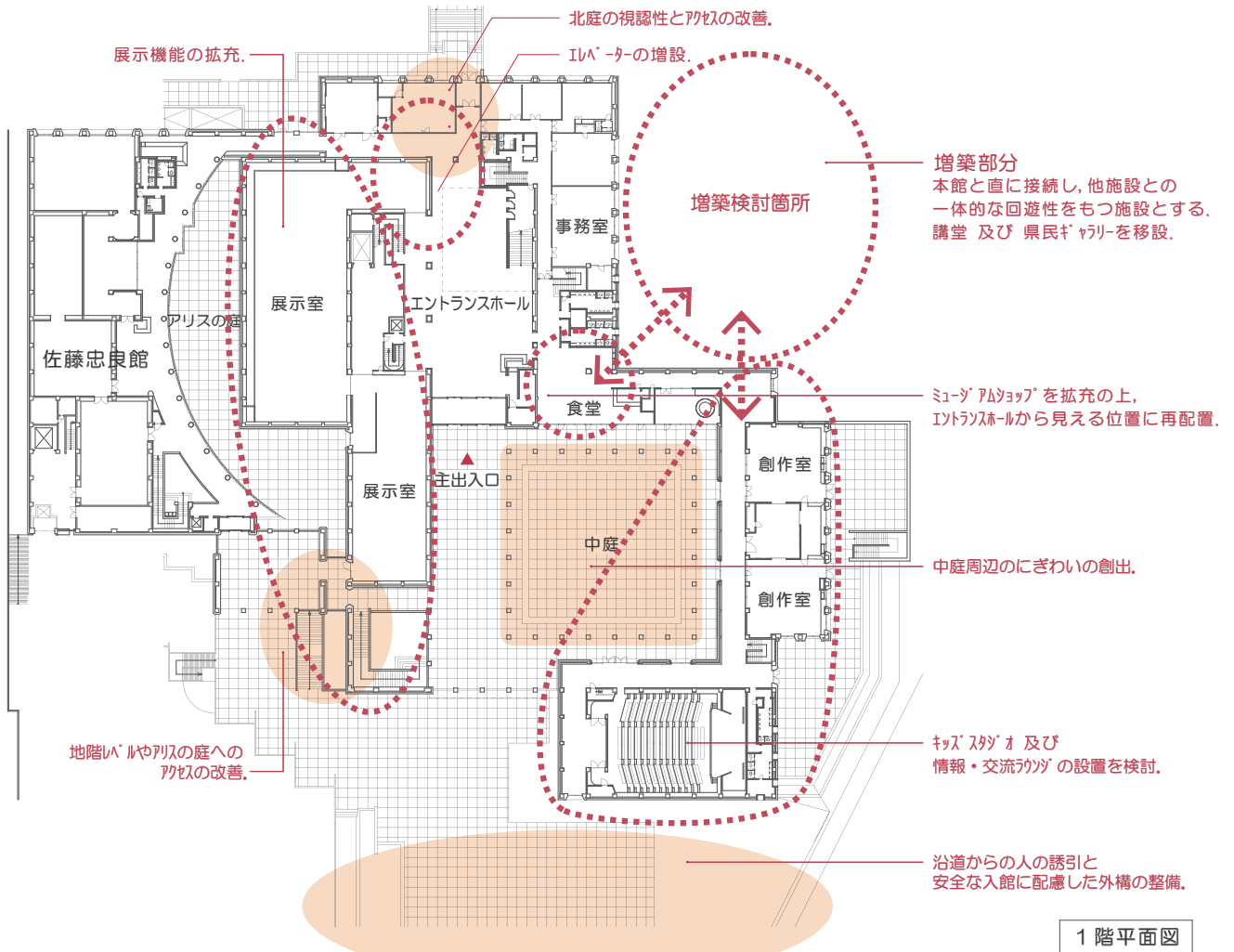
図7. 施設整備計画図
