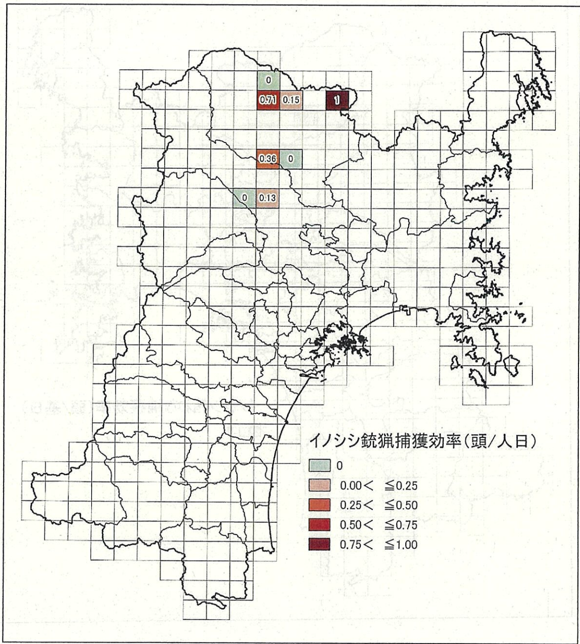
平成29年度指定管理鳥獣捕獲等事業捕獲（イノシシ）SPUE 位置図
