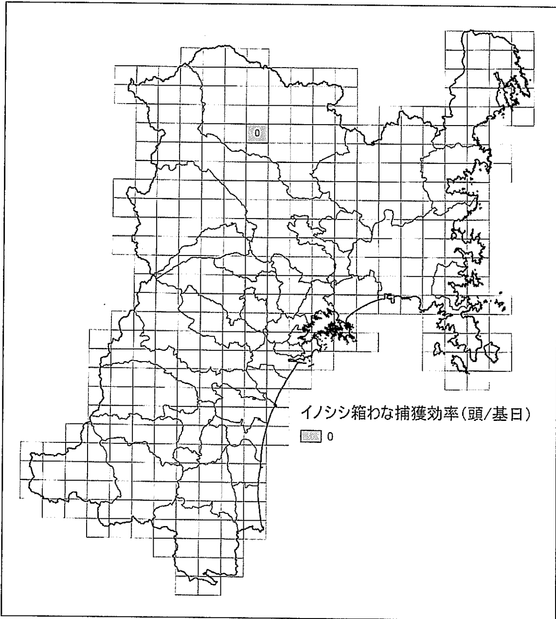
平成29年度指定管理鳥獣捕獲等事業捕獲（イノシシ）CPUE（箱わな）位置図
