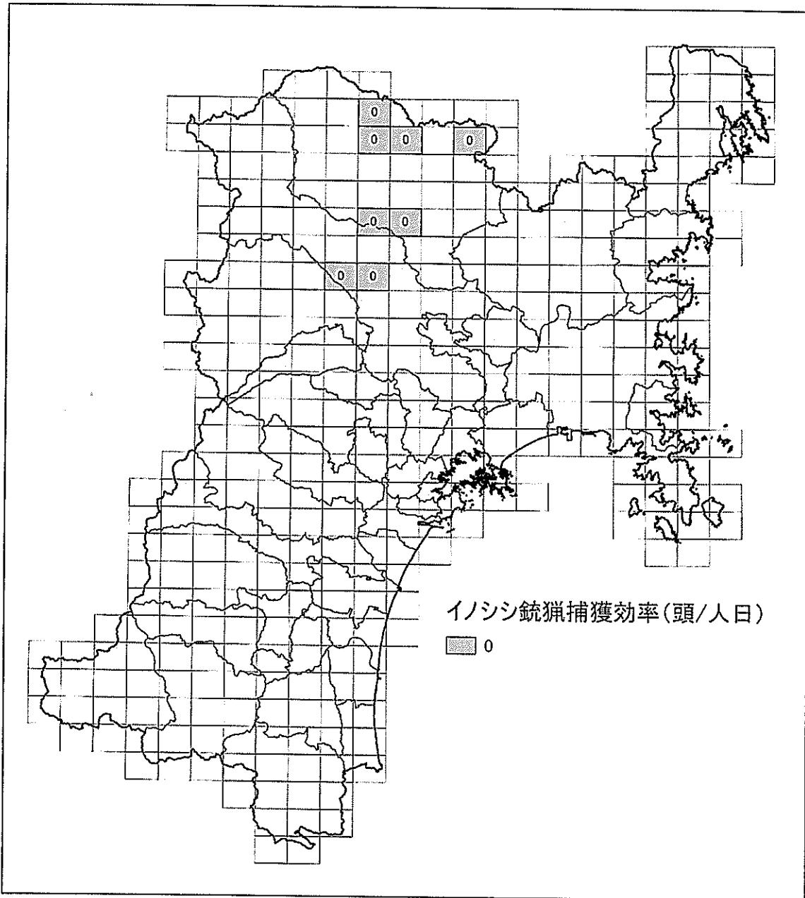
平成29年度指定管理鳥獣捕獲等事業捕獲（イノシシ）CPUE（銃）位置図
