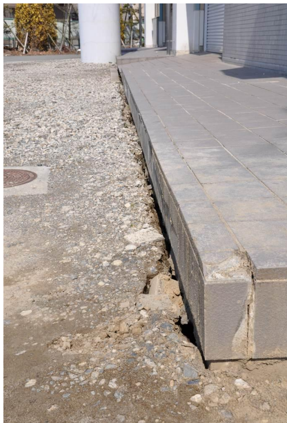
実習棟テラス付近の段差・亀裂
