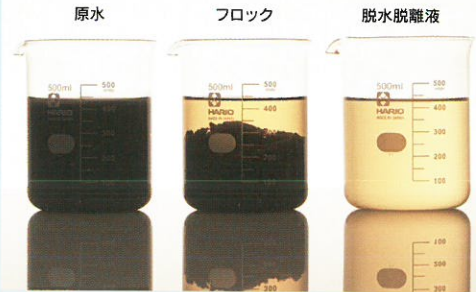
■リセルバー試験写真(余剰汚泥)
