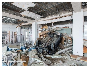
津波により被災した校舎 （写真提供：気仙沼市 東日本大震災遺構・伝承館）
