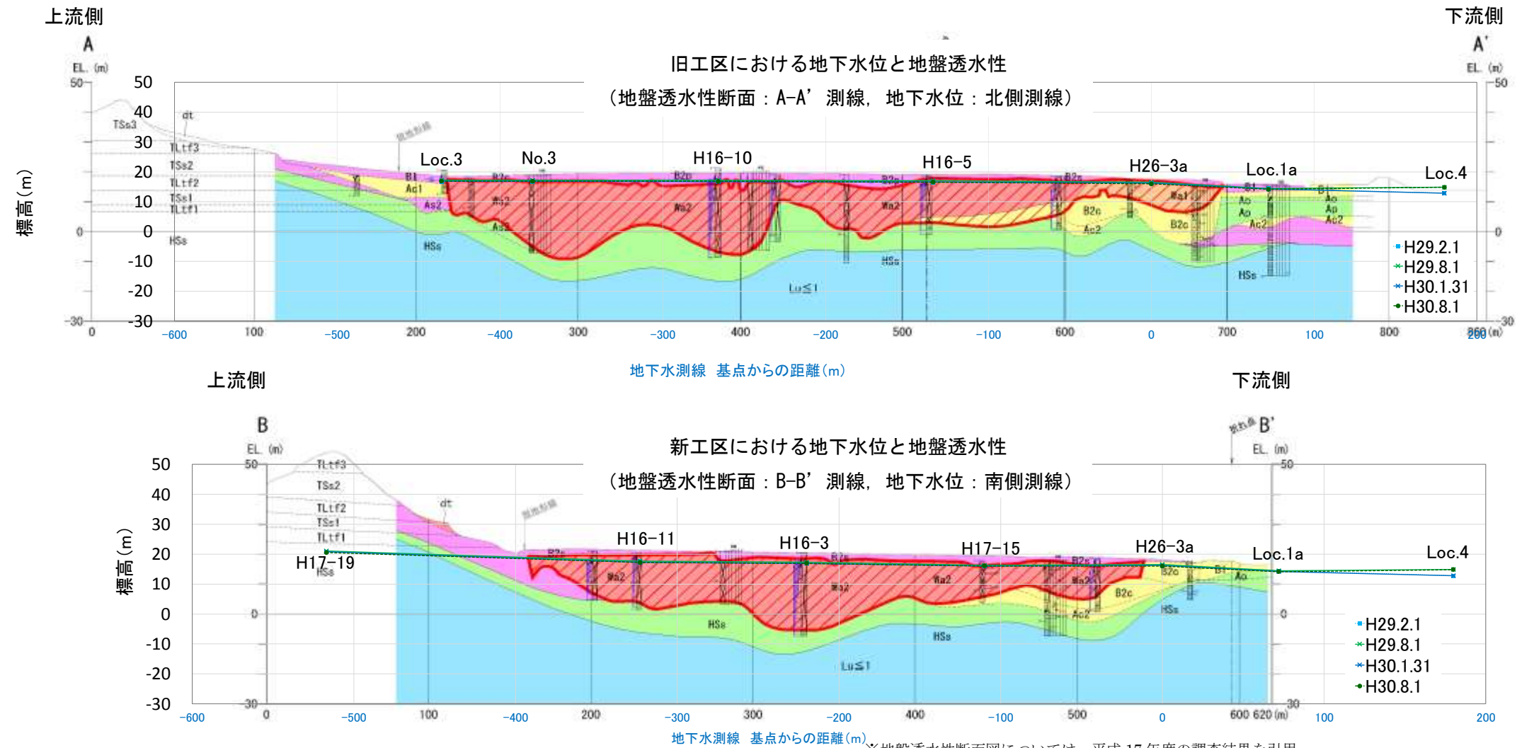
図5-13 平成30年度上期の上流側～下流側にかけての水位標高変化（地盤透水性断面図）
