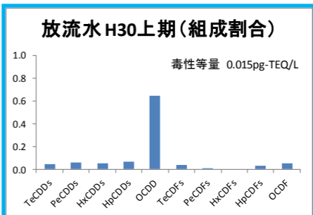
図3-2 ダイオキシン類パターン (H30上期・処分場外)
