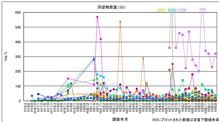
図 3-36 浮遊物質 (SS) (浸透水・地下水)
