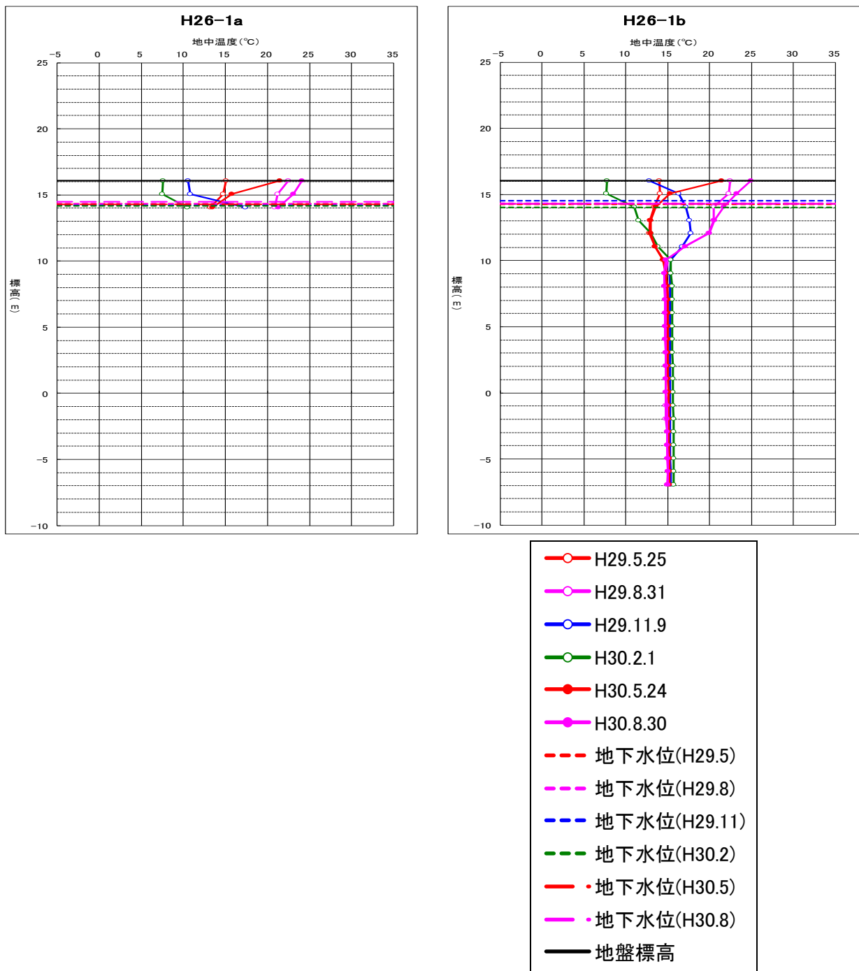
图 5-6 地中温度变化图 (地下水) ④
