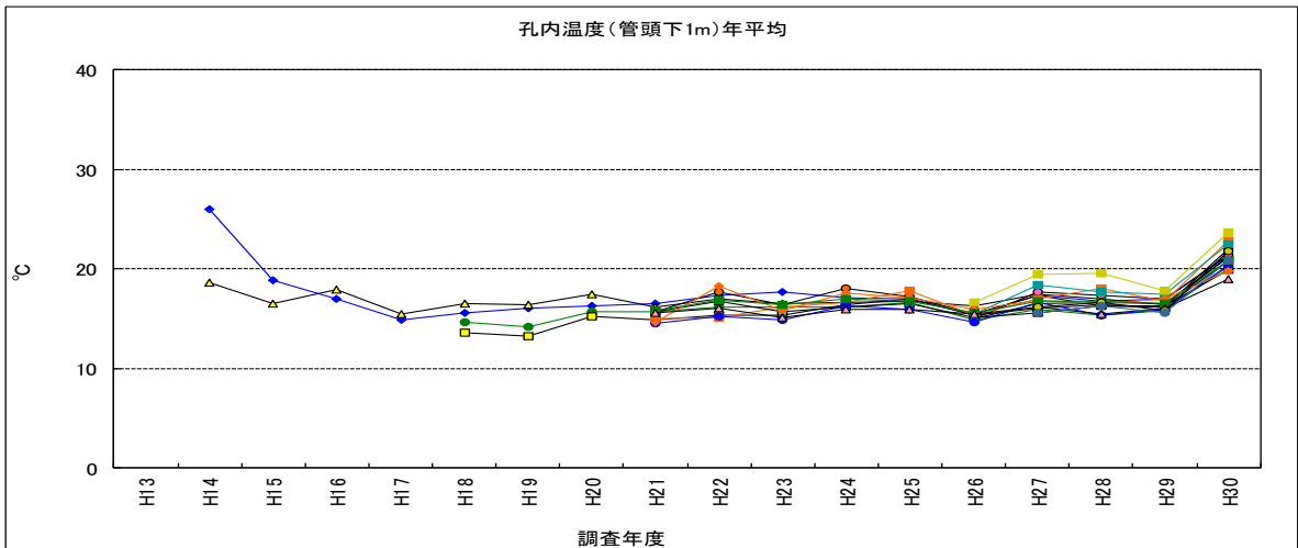
図 4-6 孔内温度 (管頭下 1m で測定)
