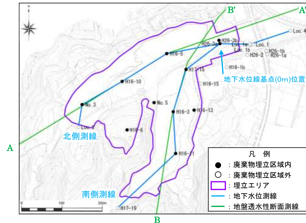
図5-14 平成30年度上期の上流側～下流側にかけての水位標高変化（平面図）
