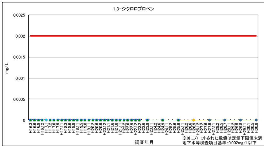
図 3-23 1,3-ジクロロプロペン (浸透水・地下水)
