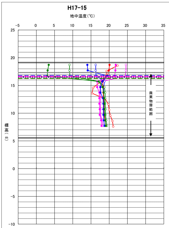
图 6-6 地中温度变化图 (浸透水) ③
