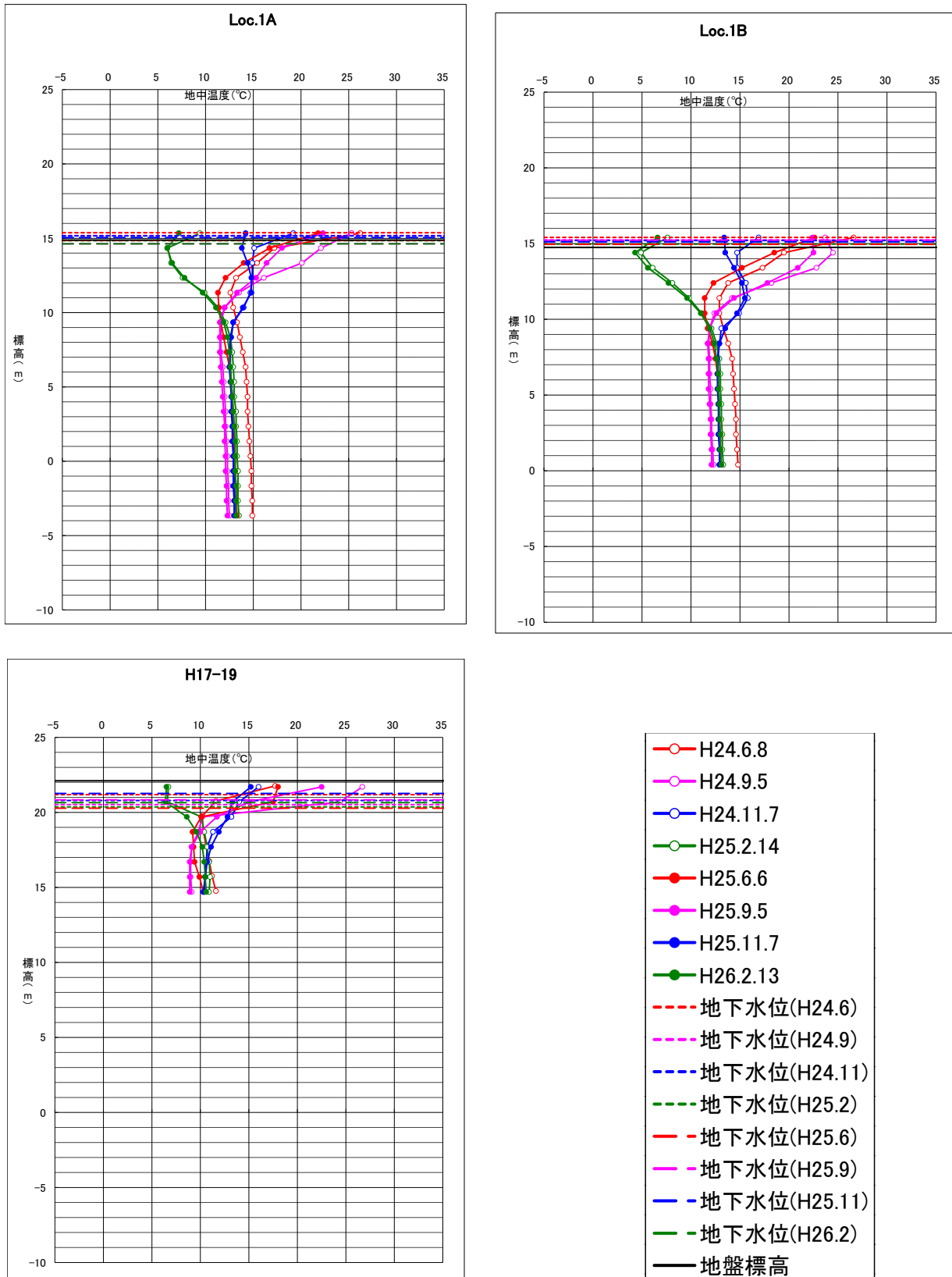
図 6-2 地中温度変化図 (地下水) ①
