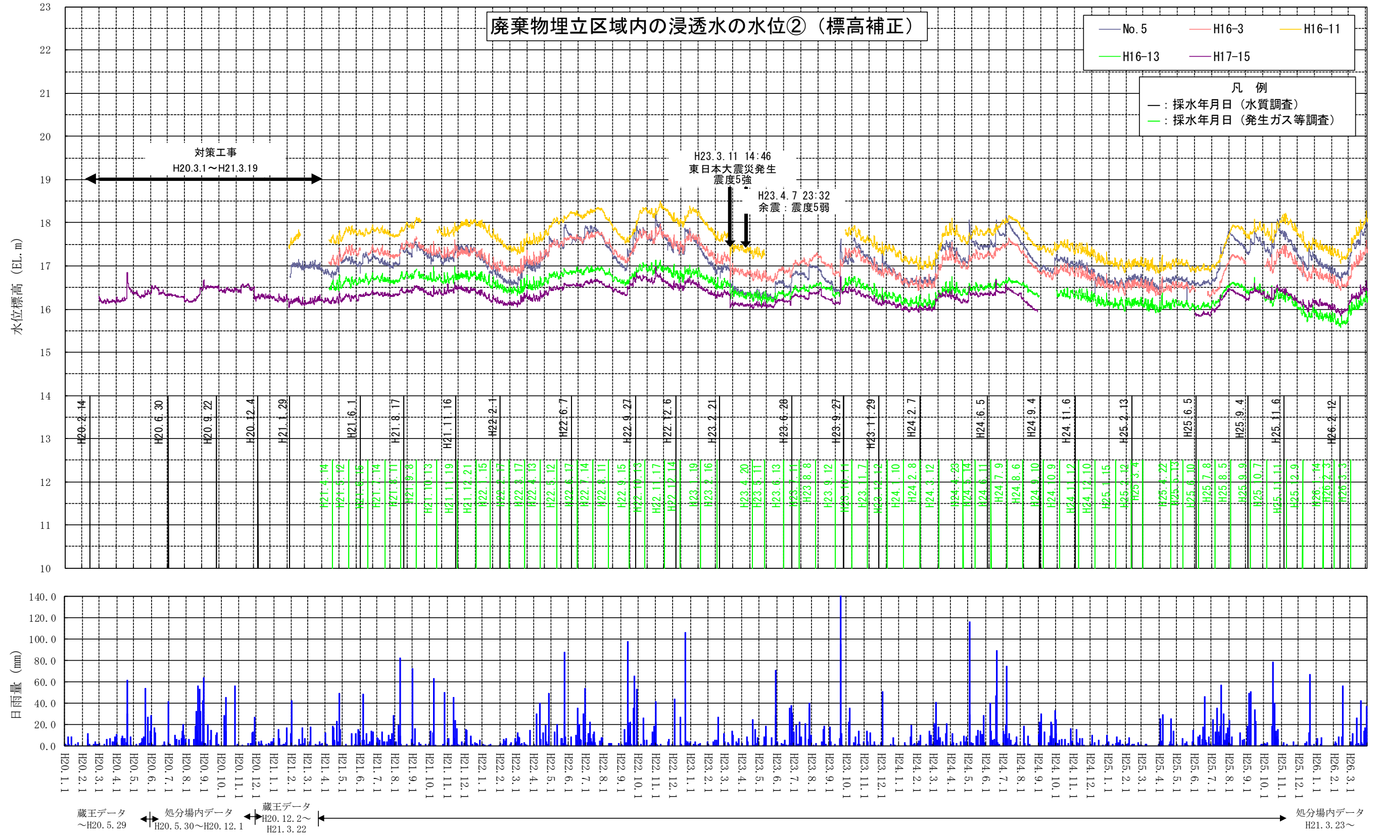
図 6-9 地下水位経時変化図 (廃棄物埋立区域内の浸透水の水位②)
