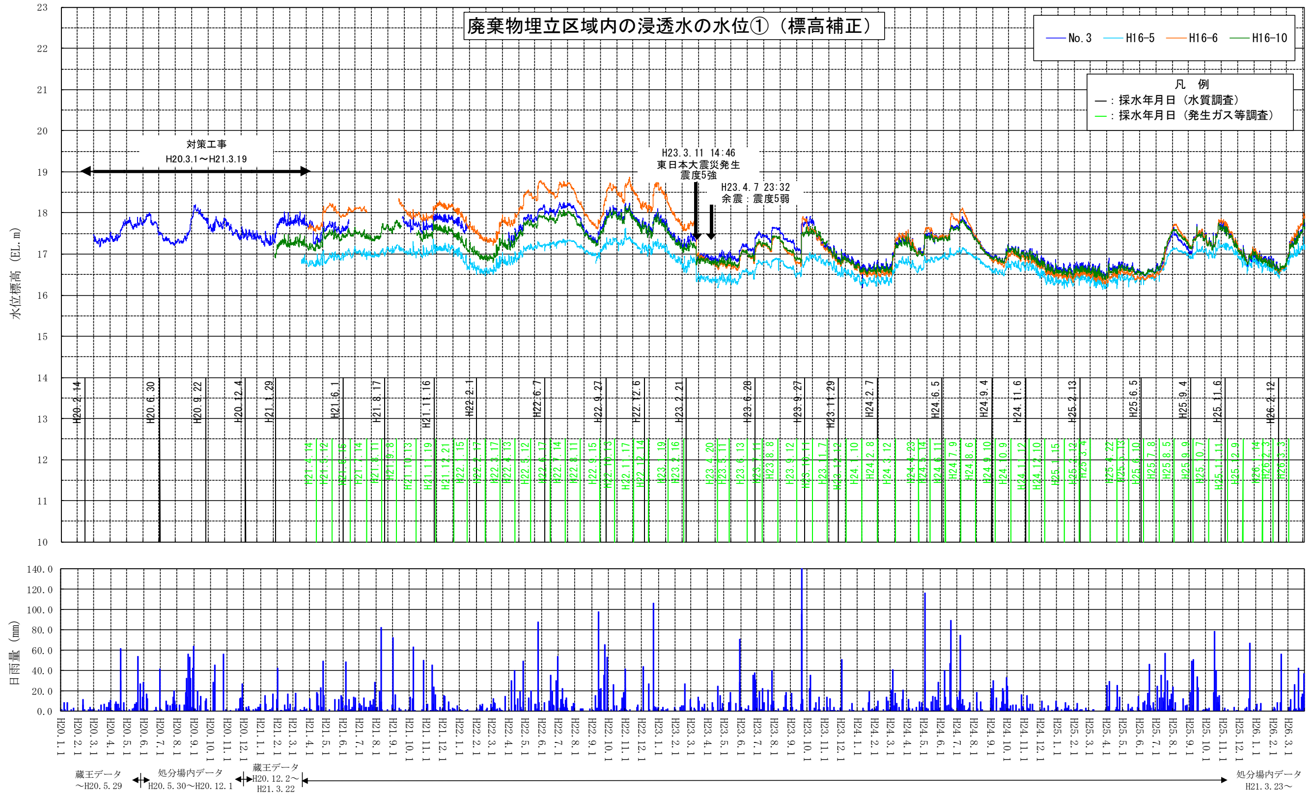
図 6-8 地下水位経時変化図 (廃棄物埋立区域内の浸透水の水位①)
