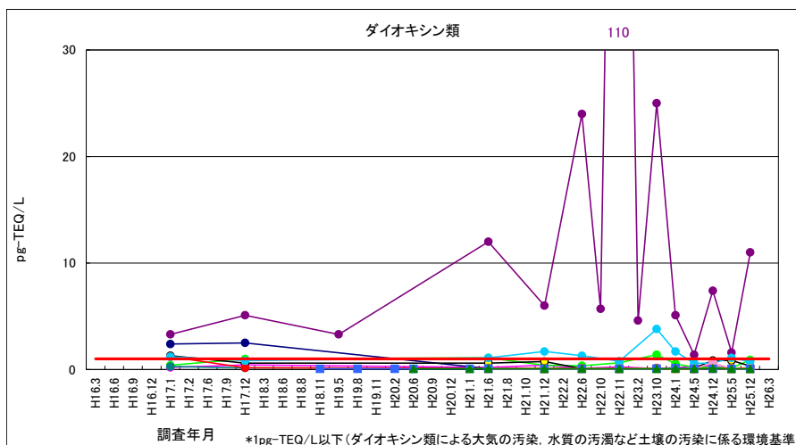
図 4-45 ダイオキシン類 (浸透水・地下水)
