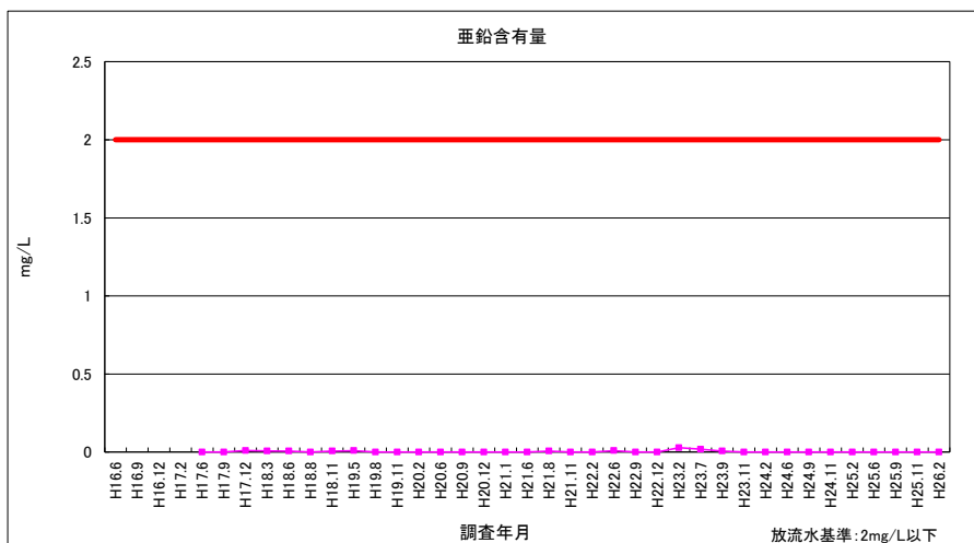
図 3-36 亜鉛含有量 (放流水)
