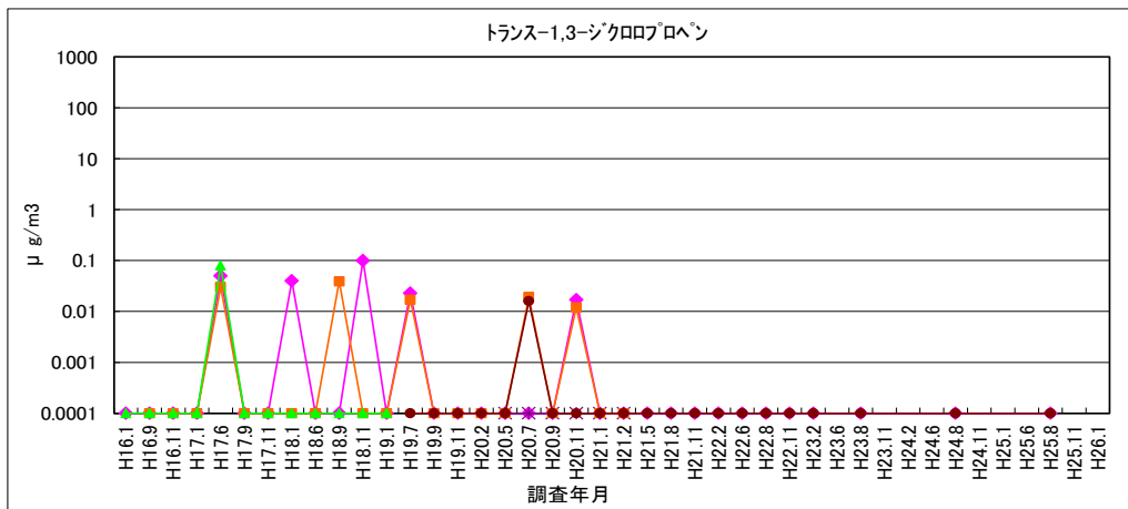
図 1-35 トランス-1,3-ジクロロプロペン
