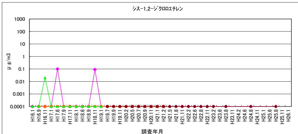
図 1-21 シス-1,2-ジクロロエチレン
