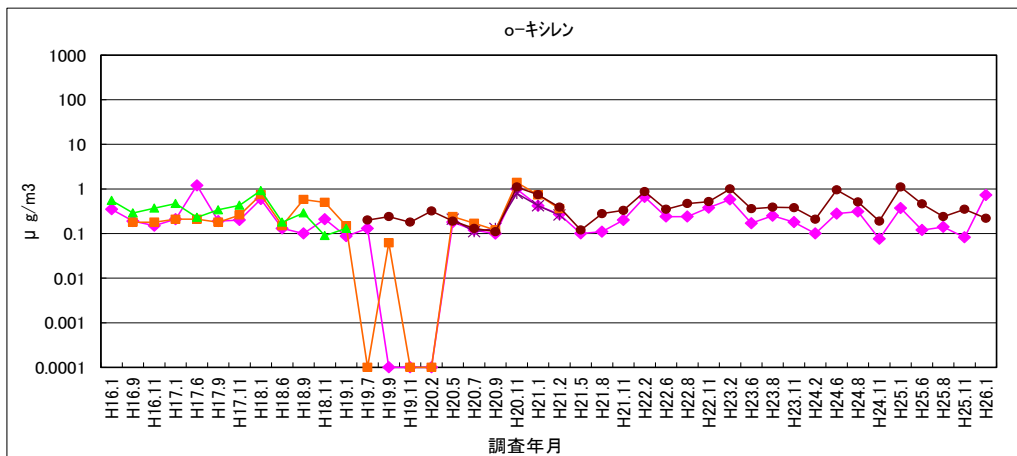
図 1-39 o-キシレン
