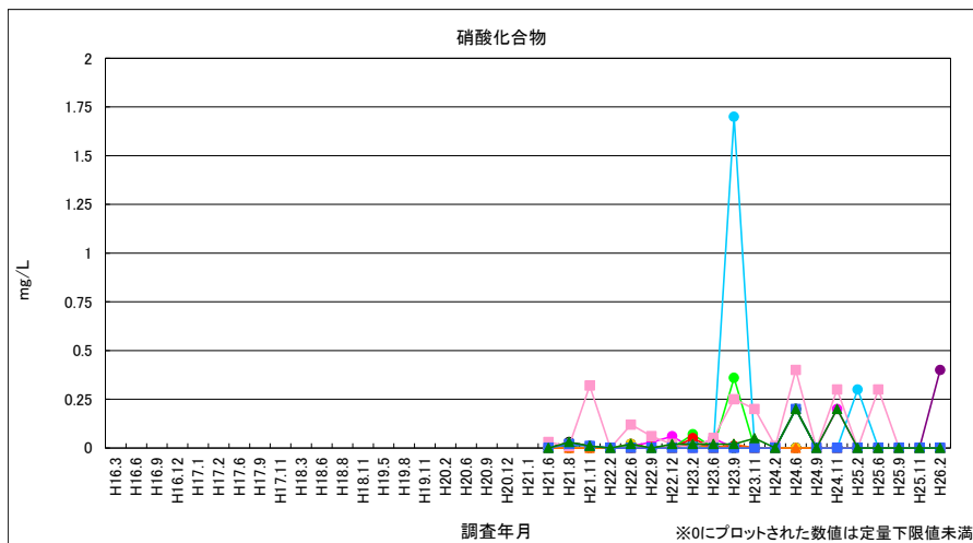
図 4-34 硝酸化合物（浸透水・地下水）
