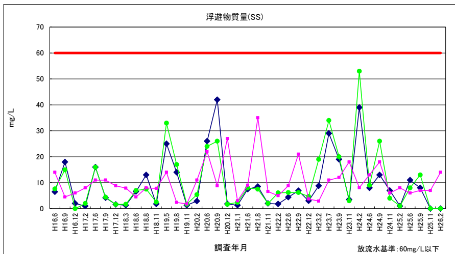
図 3-31 浮遊物質質量 (SS) (放流水・河川水)
