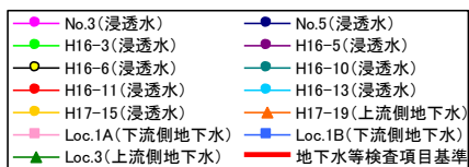
図 4-33 亜硝酸化合物 (浸透水・地下水)
