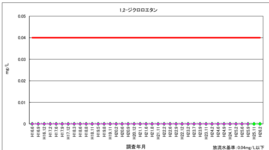
図 3-14 1,2-ジクロロエタン（放流水・河川水）
