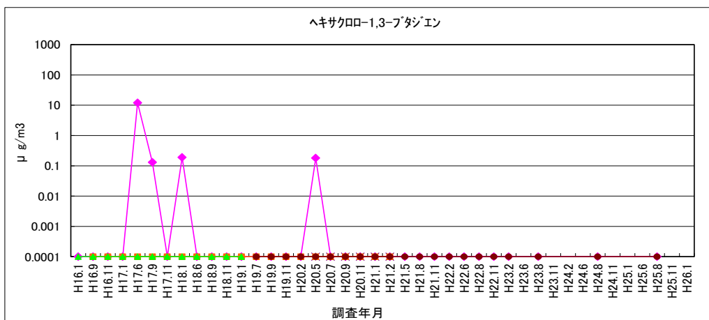
図 1-48 ヘキサクロロ-1,3-ブタジエン
