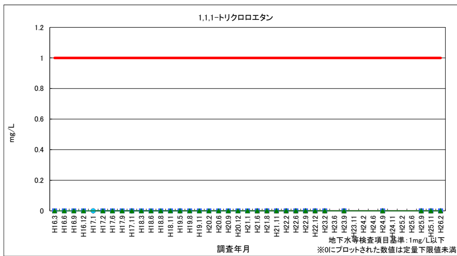
図 4-17 1,1,1-トリクロロエタン (浸透水・地下水)
