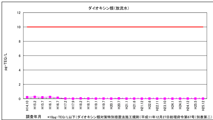
図 3-49 ダイオキシン類 (放流水)
