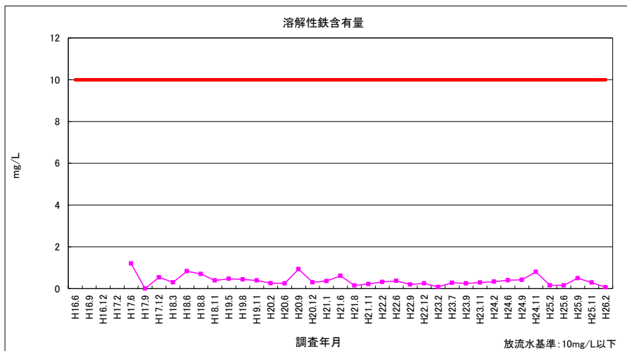
図 3-37 溶解性鉄含有量 (放流水)
