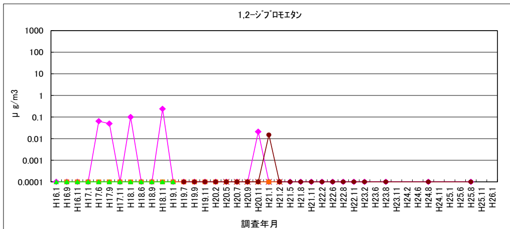
図 1-36 1,2-ジブロモエタン
