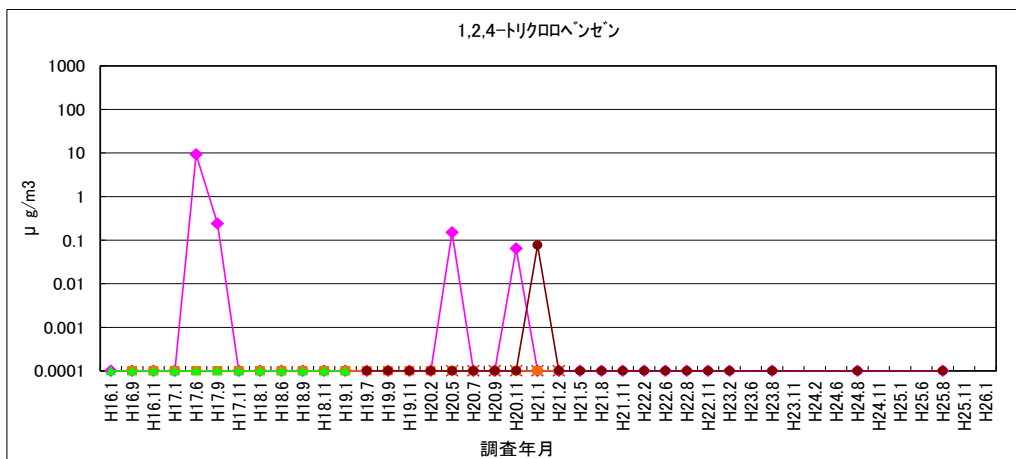
図 1-47 1,2,4-トリクロロベンゼン
