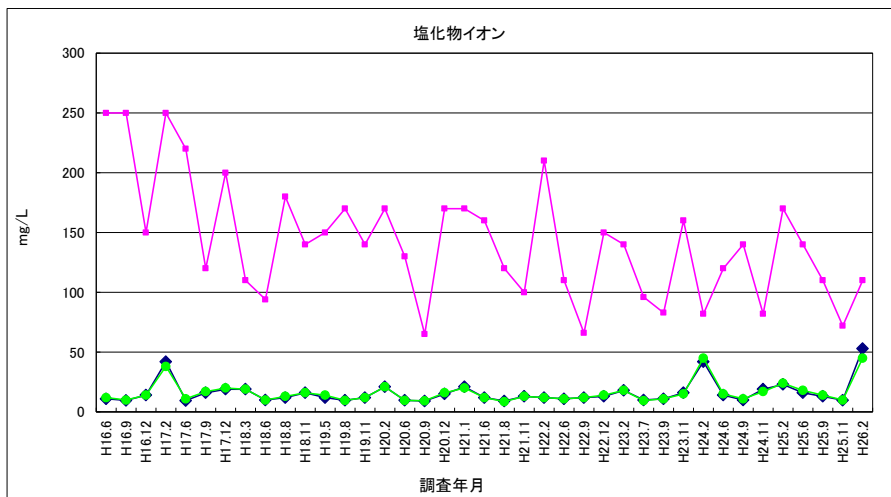
図 3-43 塩化物イオン（放流水・河川水）
