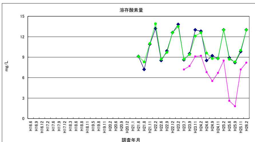
図 3-41 溶存酸素量 (河川水・放流水)
