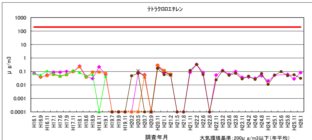
図 1-15 テトラクロロエチレン
