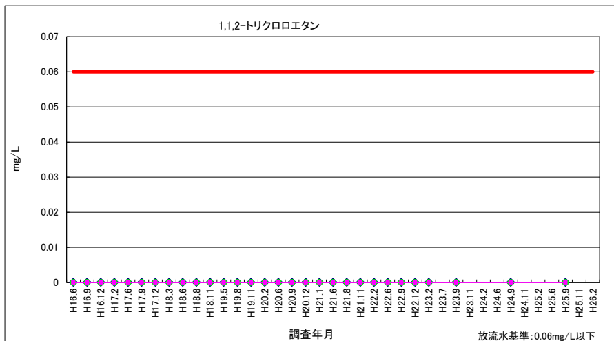
図 3-18 1,1,2-トリクロロエタン (放流水・河川水)
