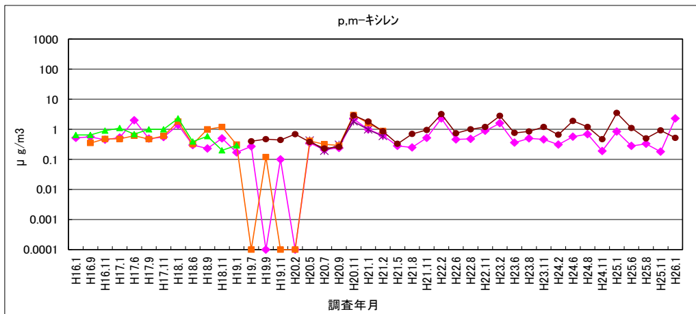
図 1-38 p, m-キシレン
