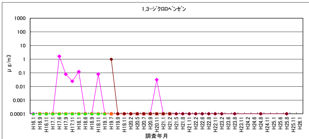
図 1-44 1,3-ジクロロベンゼン
