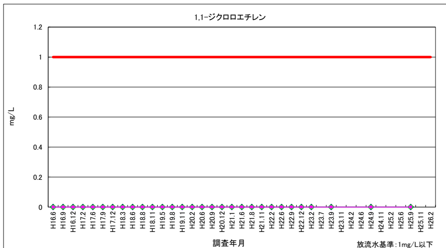
図 3-15 1,1-ジクロロエチレン（放流水・河川水）
