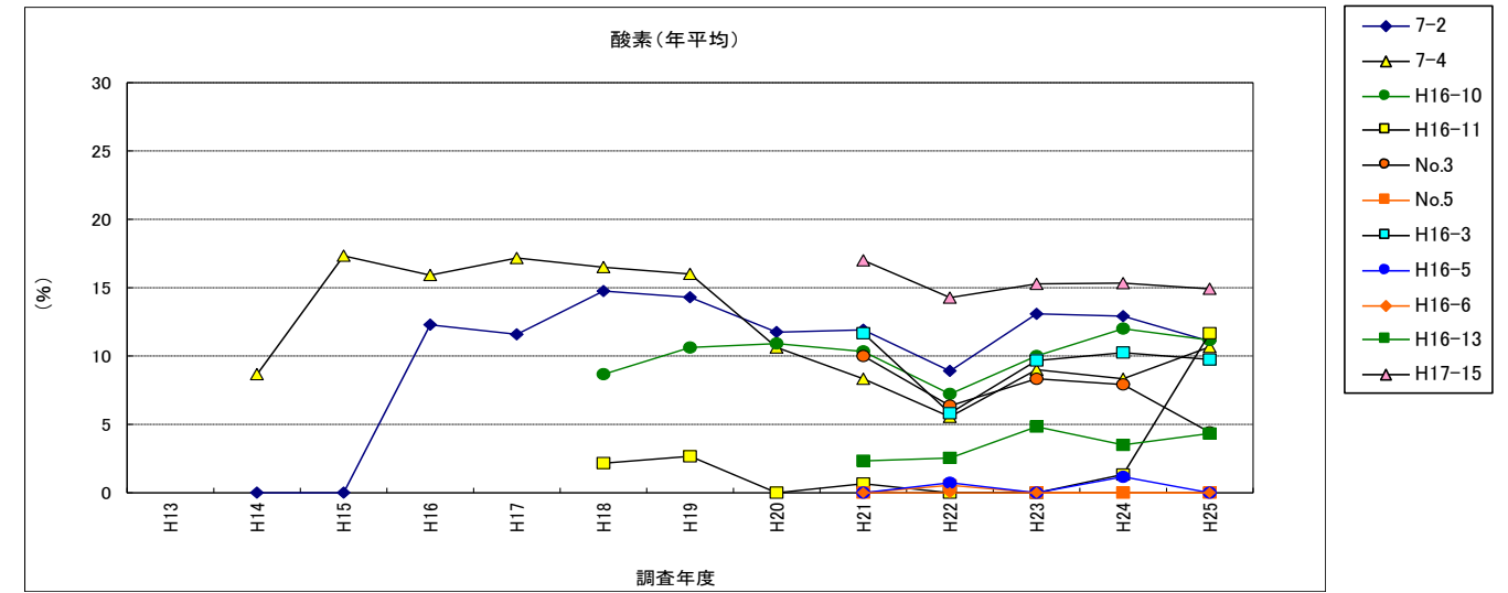
図 5-3 酸素 (管頭下 1 m で測定)
