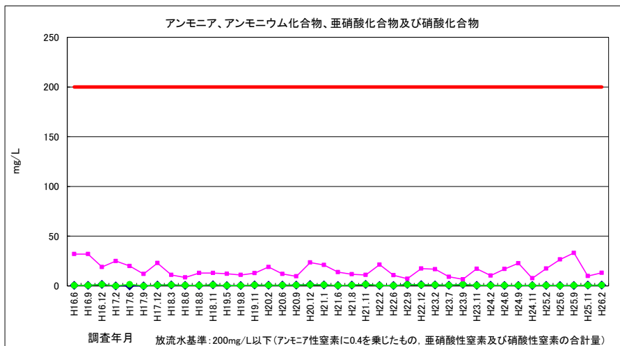
図 3-28 アンモニア、アンモニア化合物、亜硝酸化合物及び硝酸化合物（放流水・河川水）
