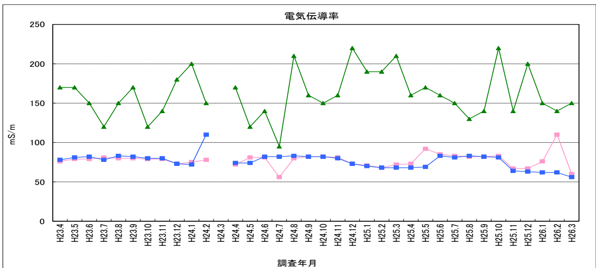
図 5-13 電気伝導率
