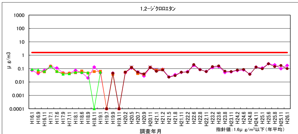
図 1-12 1,2-ジクロロエタン
