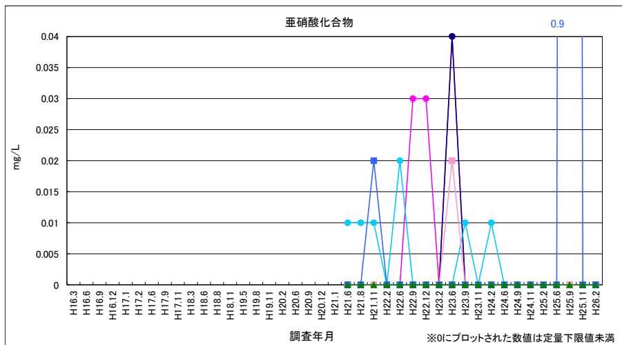
図 4-33 亜硝酸化合物 (浸透水・地下水)
