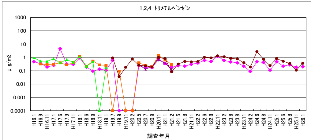
図 1-43 1,2,4-トリメチルベンゼン
