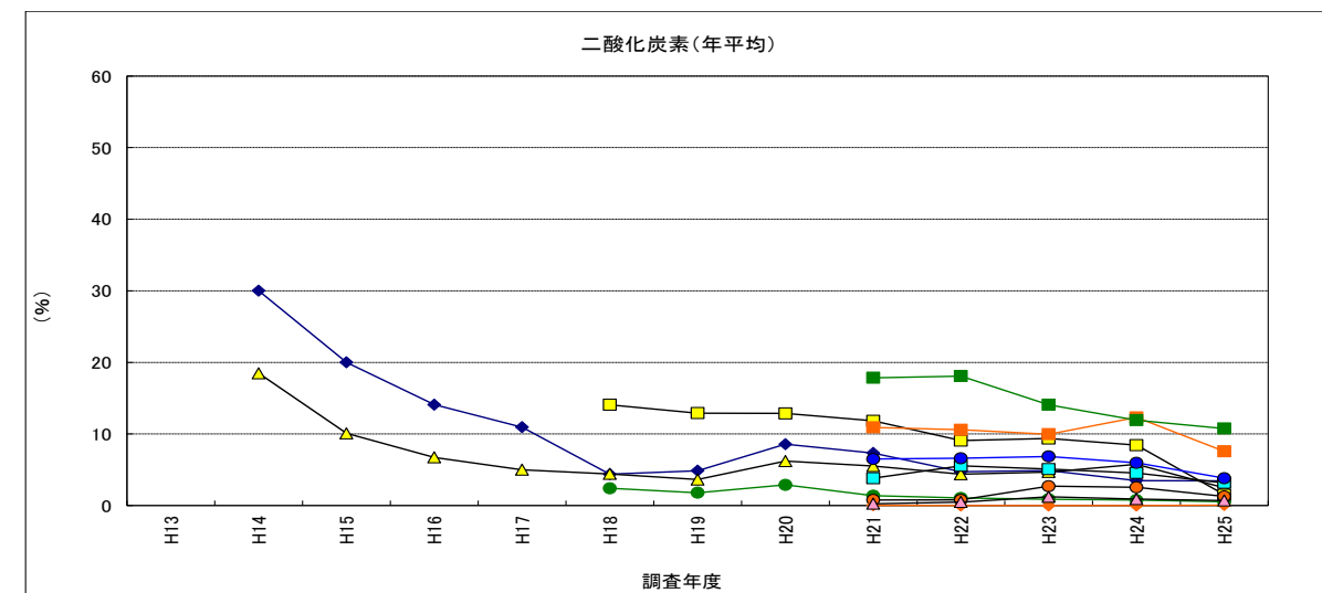
図 5-2 二酸化炭素（管頭下 1 m で測定）
