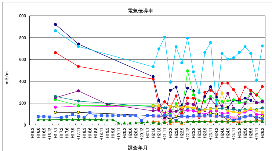
図 4-43 電気伝導率 (浸透水・地下水)
