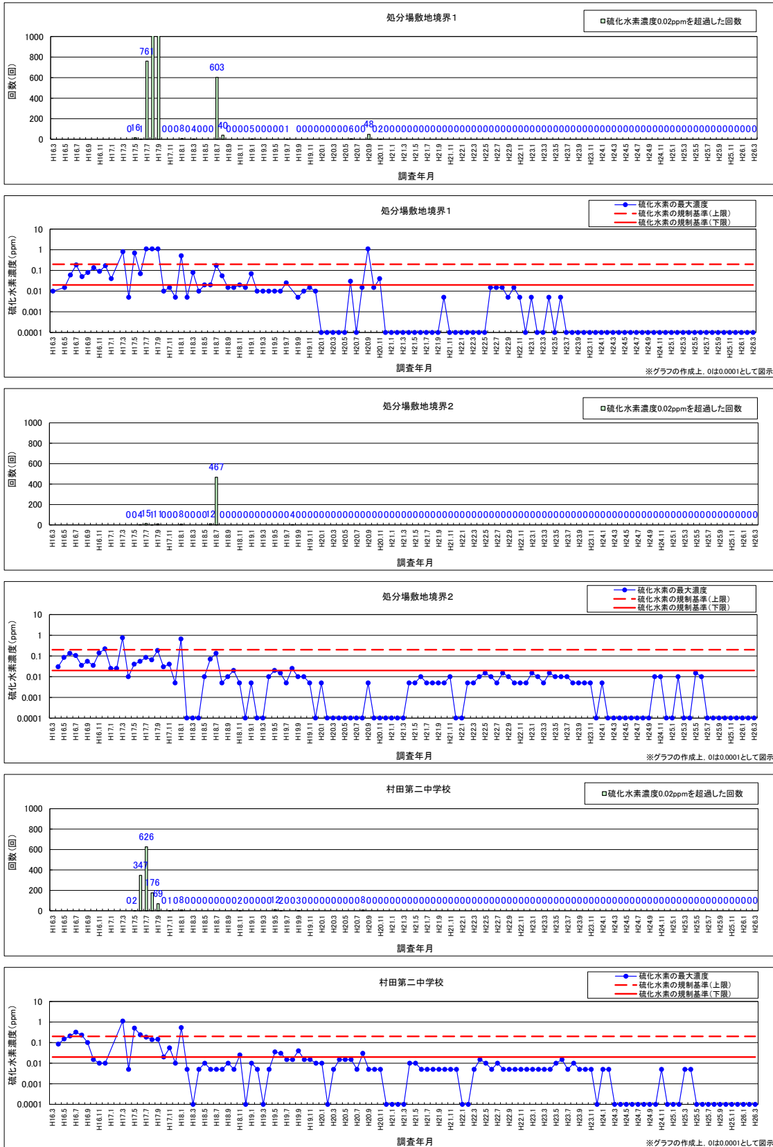
図 2-1 硫化水素連続調査結果図
