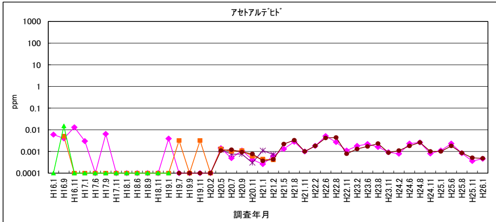
図 1-16 アセトアルデヒド
