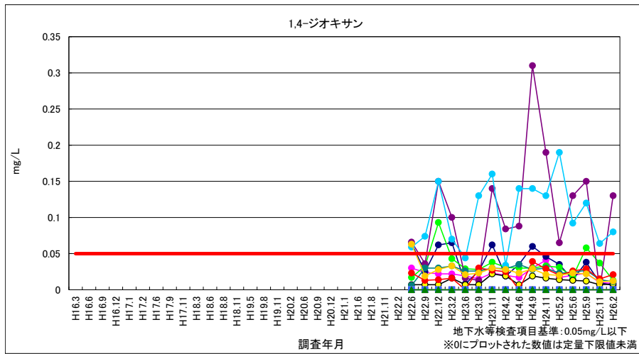
図 4-25 1,4-ジオキサン (浸透水・地下水)
