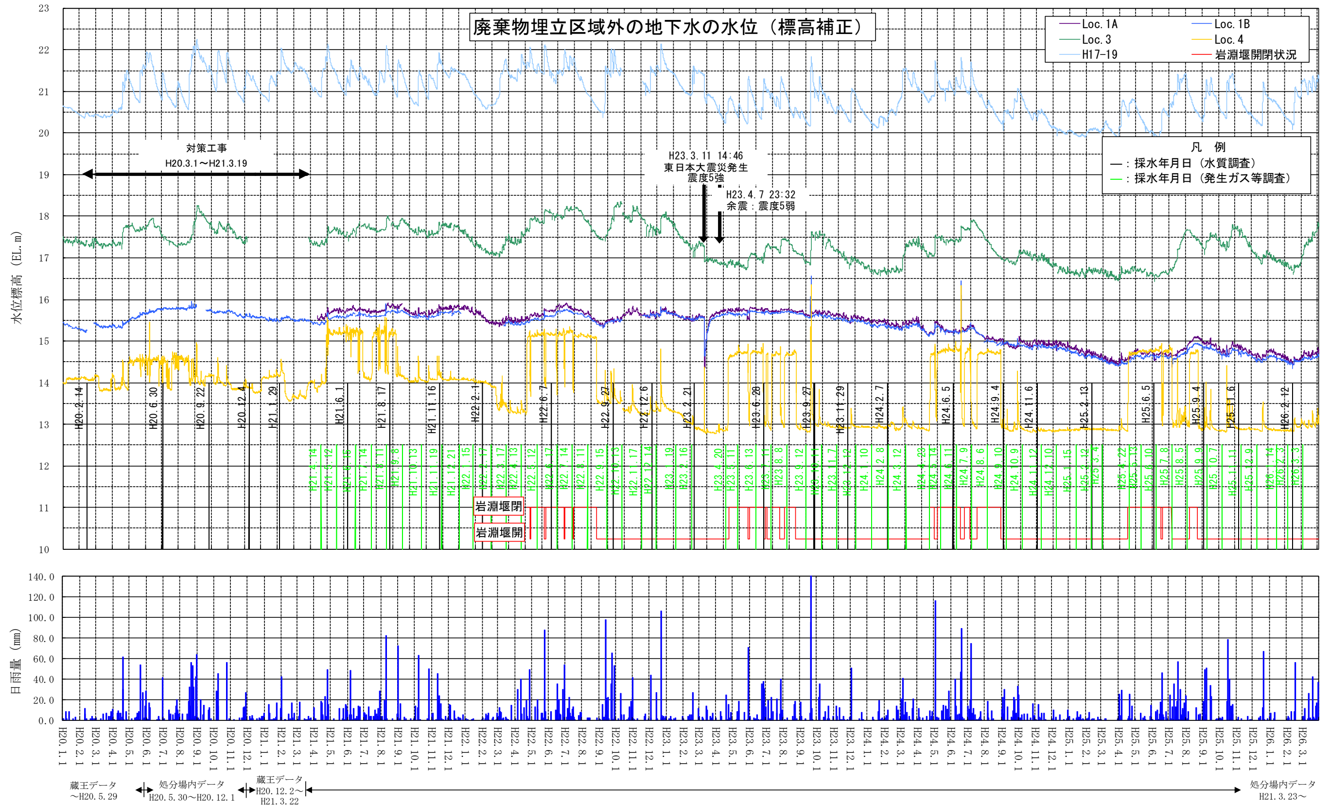
図 6-7 地下水位経時変化図（廃棄物埋立区域外の地下水の水位）
