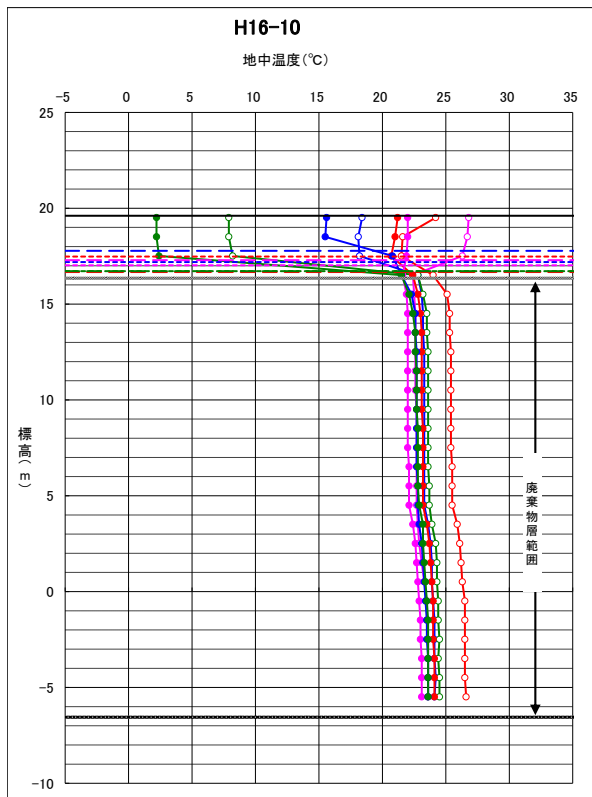
图 6-5 地中温度变化图 (浸透水) ②
