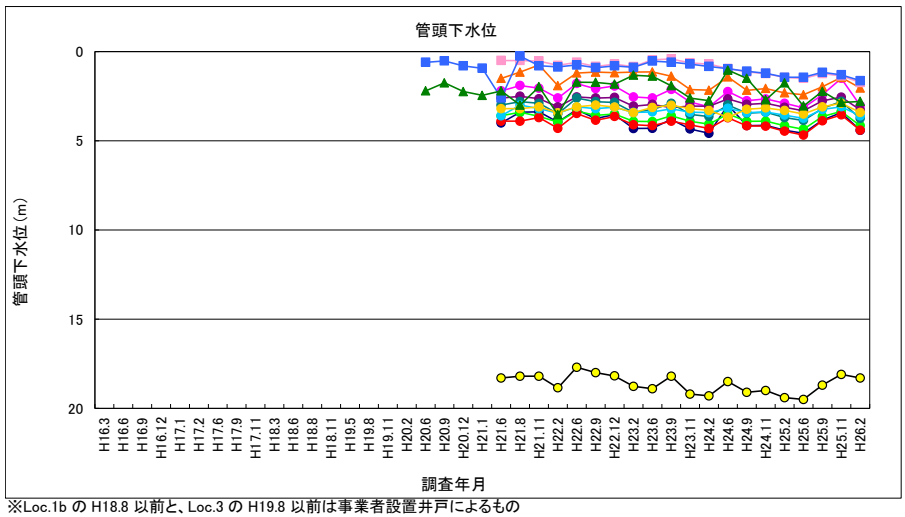
図 4-42 管頭下水位（浸透水・地下水）
