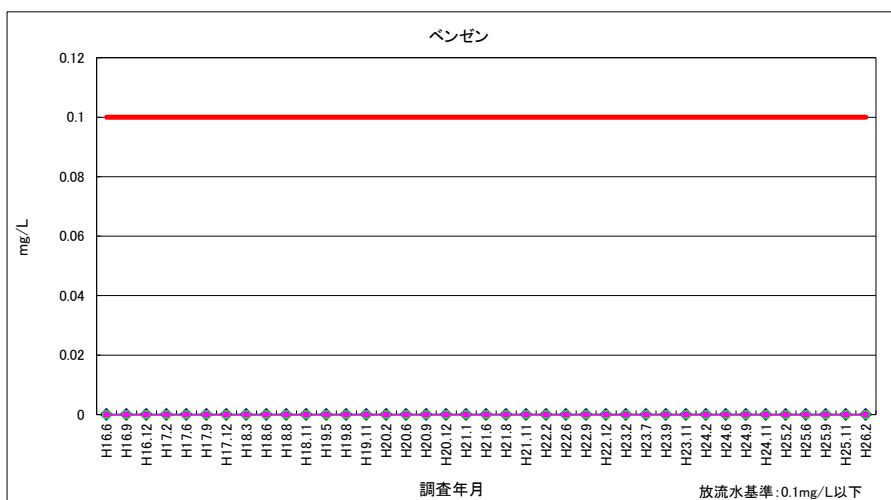
図 3-23 ベンゼン（放流水・河川水）
