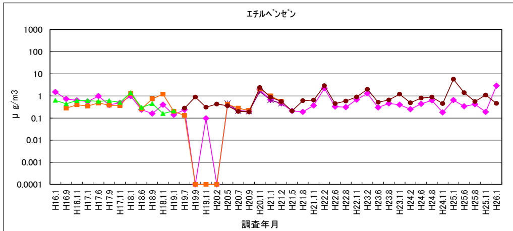
図 1-37 エチルベンゼン
