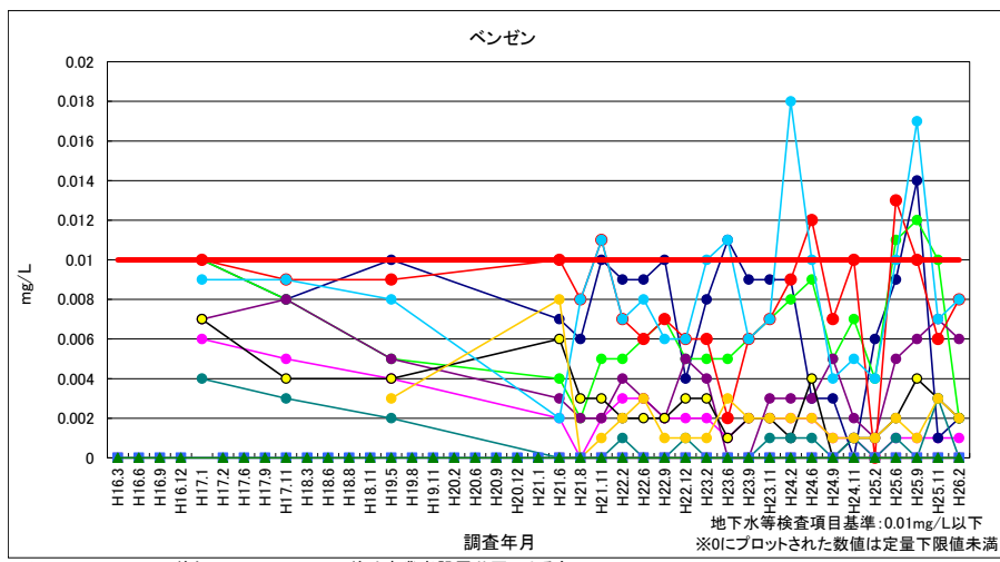
図 4-23 ベンゼン（浸透水・地下水）
