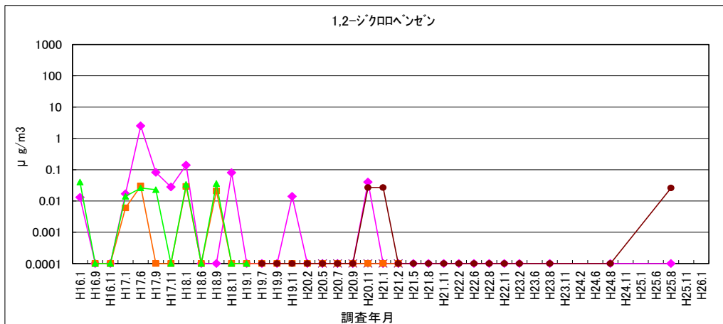
図 1-46 1,2-ジクロロベンゼン
