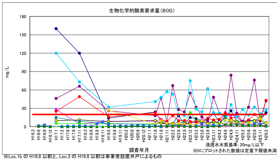
図 4-27 生物化学的酸素要求量 (BOD) (浸透水・地下水)
