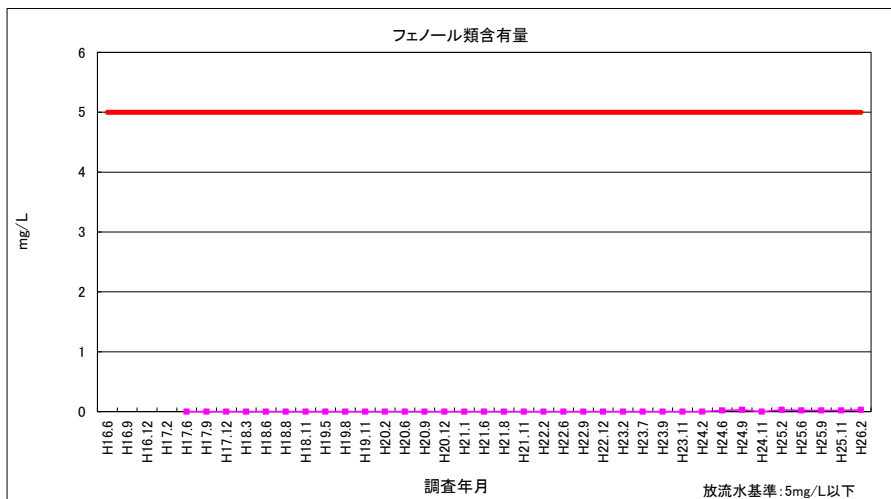
図 3-34 フェノール類含有量 (放流水)
