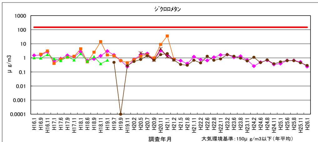
図 1-9 ジクロロメタン
