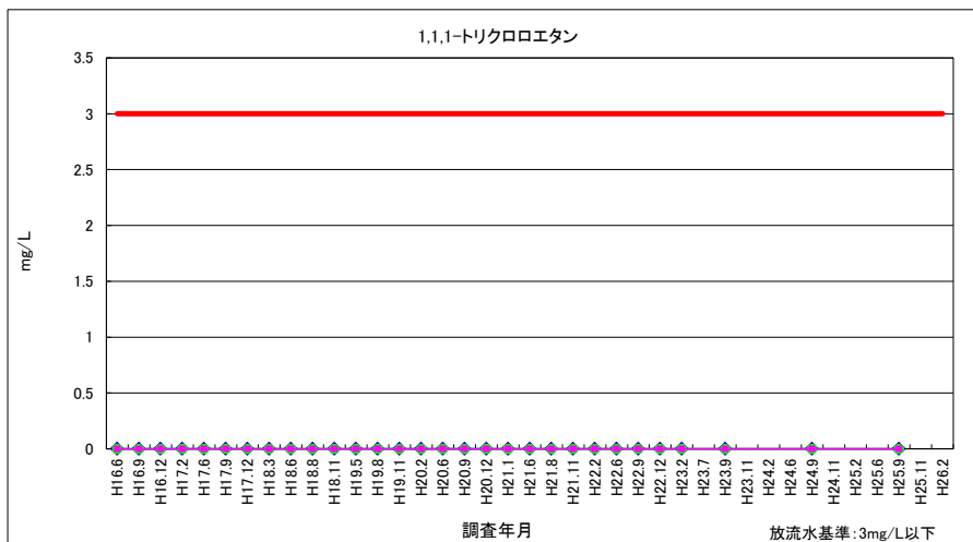
図 3-17 1,1,1-トリクロロエタン (放流水・河川水)
