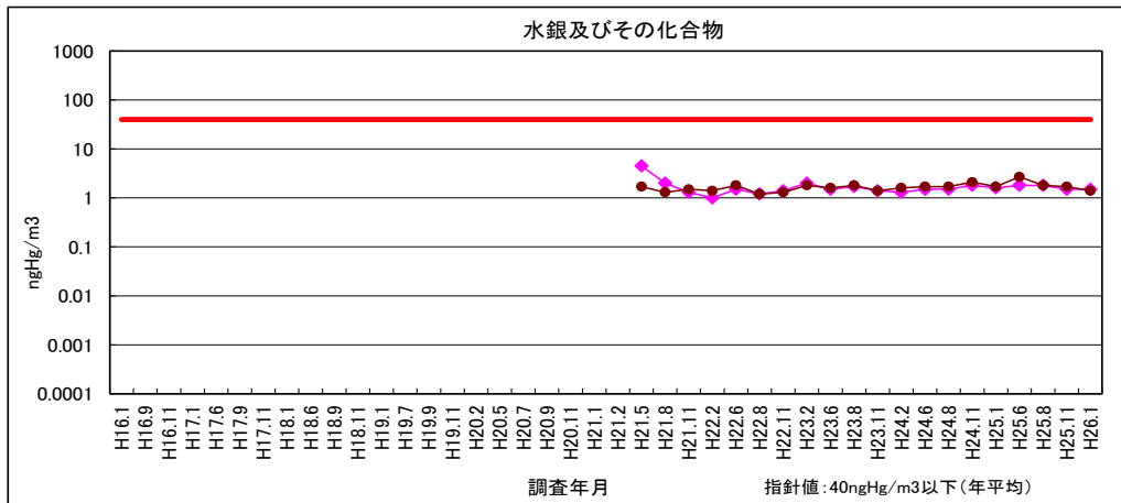
図 1-17 水銀及びその化合物
