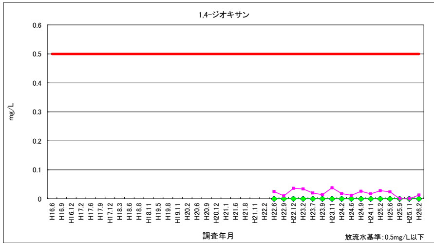
図 3-25 1,4-ジオキサン (放流水・河川水)
