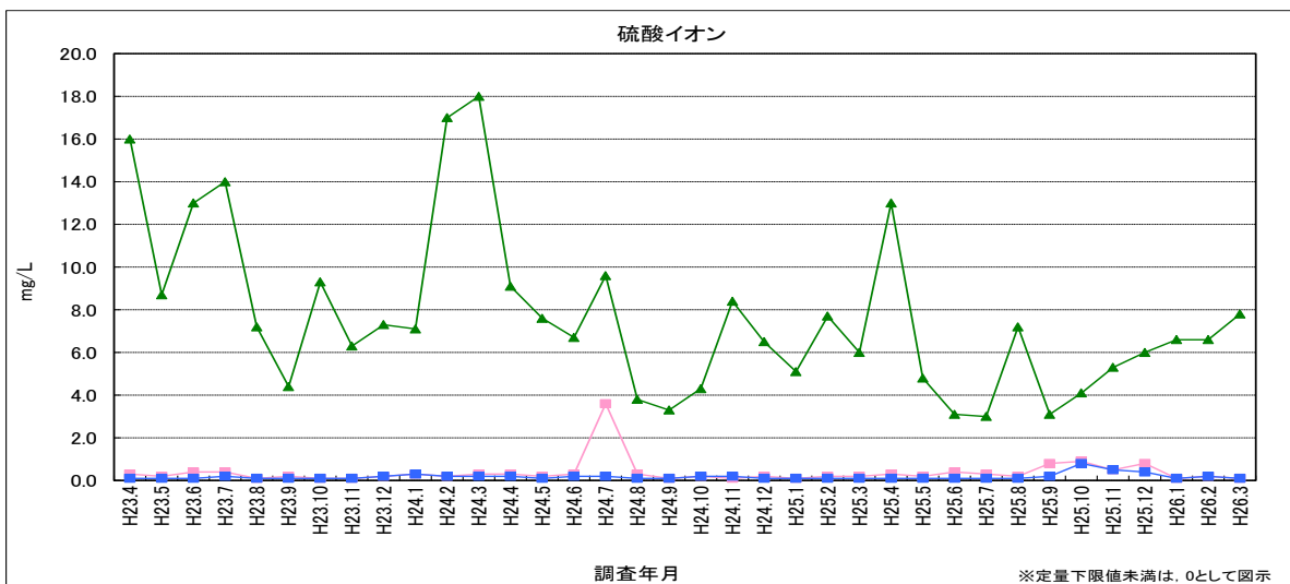
図 5-11 硫酸イオン
