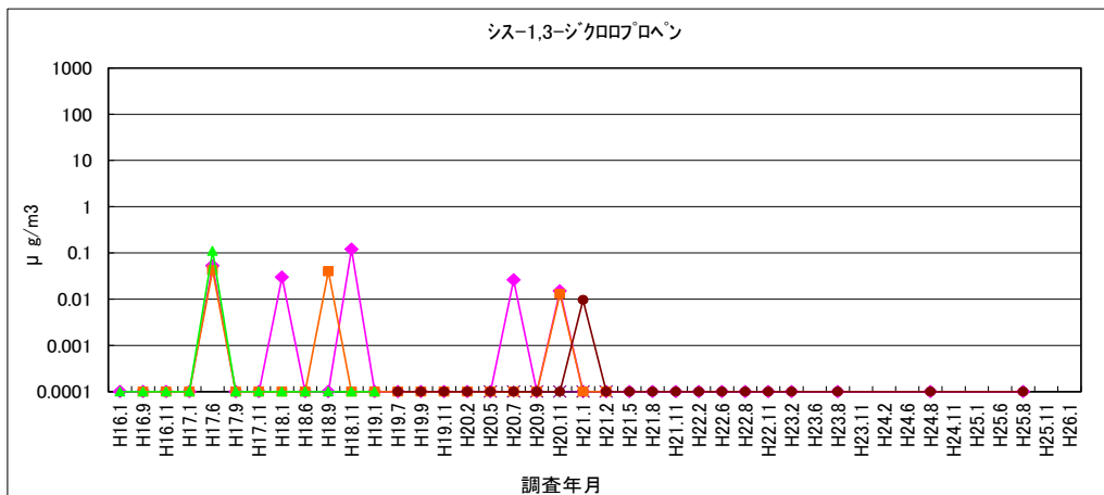
図 1-33 シス-1,3-ジクロロプロペン
