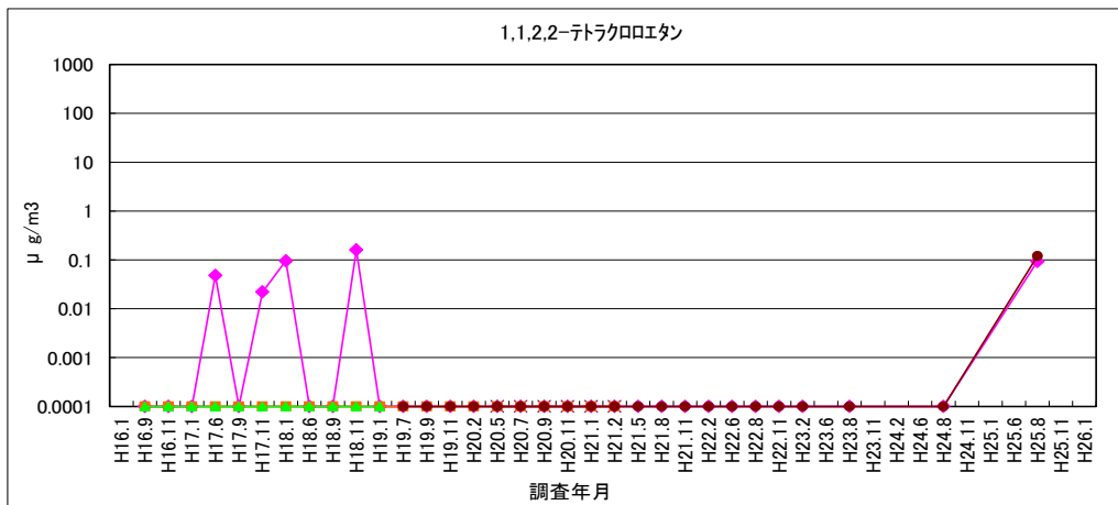
図 1-41 1,1,2,2-テトラクロロエタン
