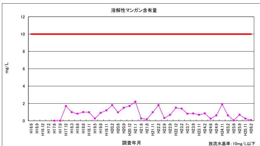
図 3-38 溶解性マンガン含有量 (放流水)
