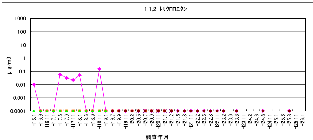
図 1-24 1,1,2-トリクロロエタン
