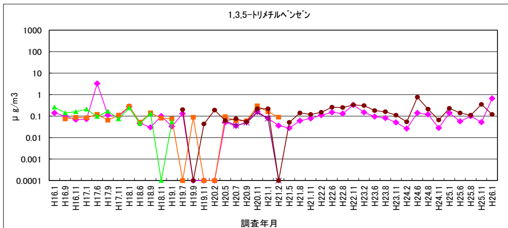
図 1-42 1,3,5-トリメチルベンゼン
