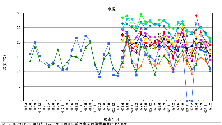
図 4-40 水温（浸透水・地下水）
