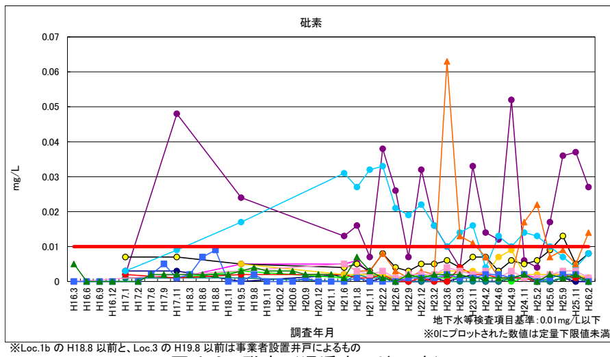
図 4-6 砒素 (浸透水・地下水)
