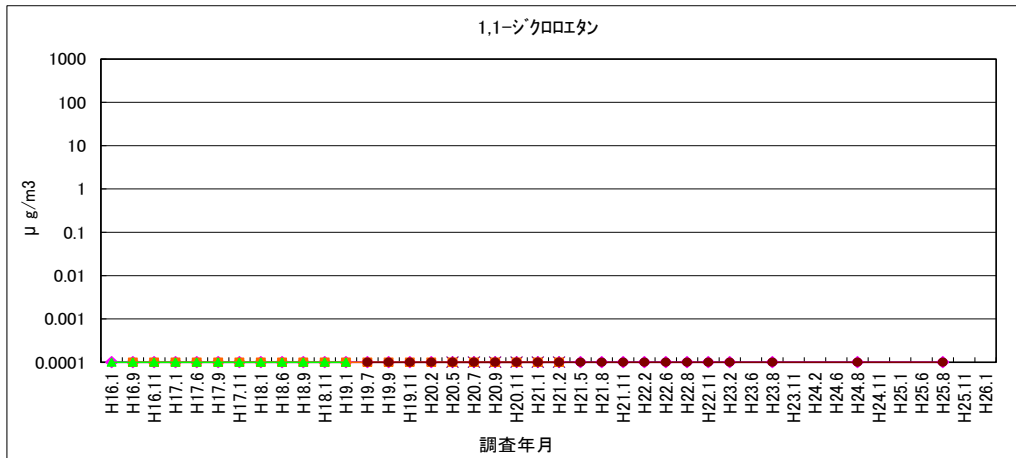
図 1-31 1,1-ジクロロエタン
