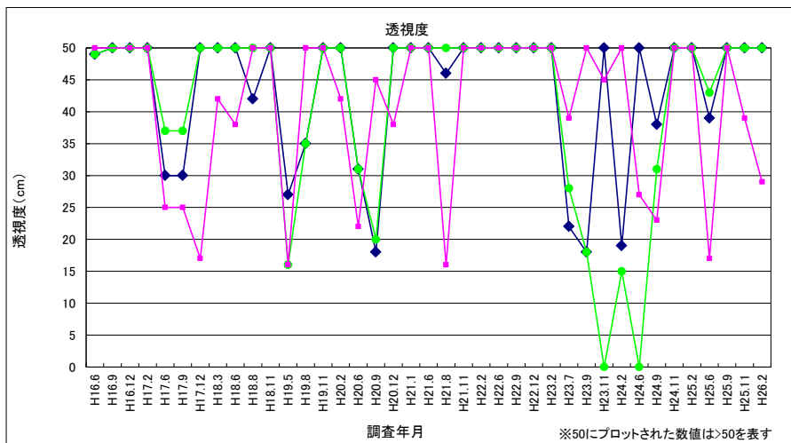
図 3-46 透視度 (放流水・河川水)
