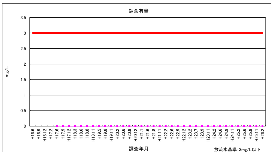
図 3-35 銅含有量 (放流水)
