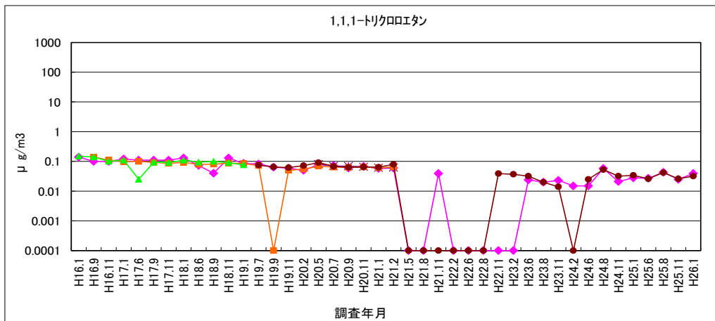
図 1-23 1,1,1-トリクロロエタン
