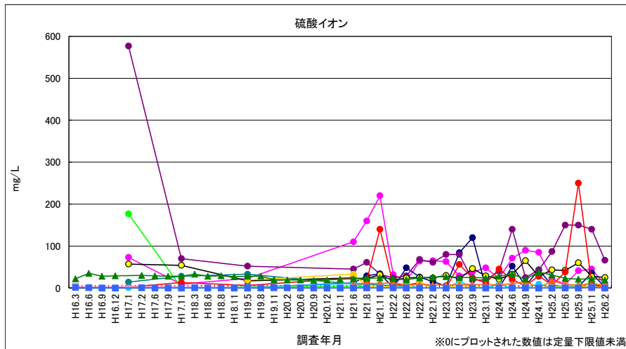
図 4-37 硫酸イオン（浸透水・地下水）
