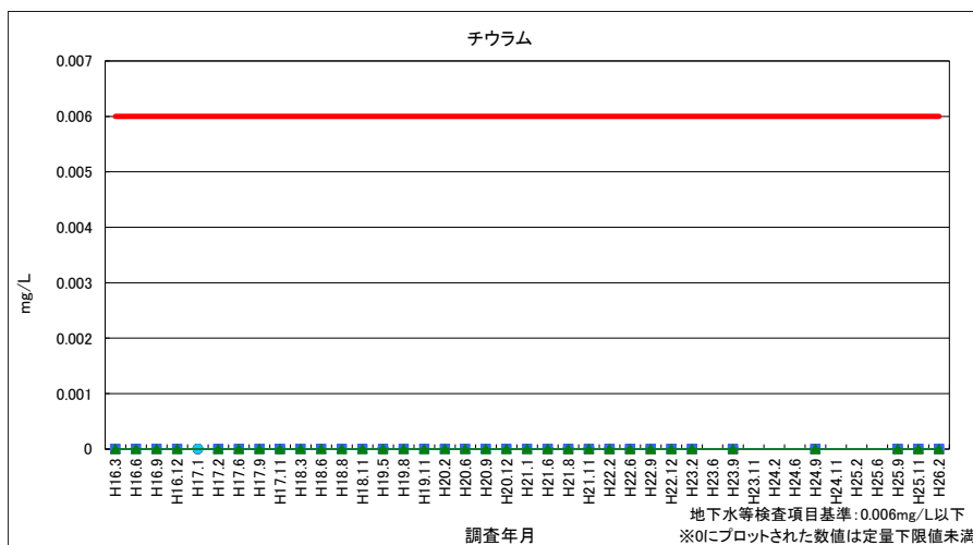
図 4-20 チウラム (浸透水・地下水)
