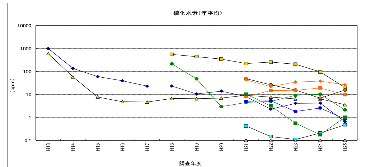
図 5-1 硫化水素（管頭下 1 m で測定）※対数表示
