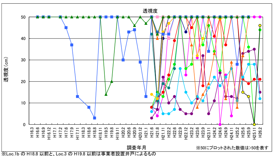
図 4-41 透視度（浸透水・地下水）
