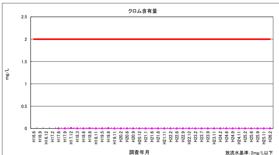
図 3-39 クロム含有量 (放流水)
