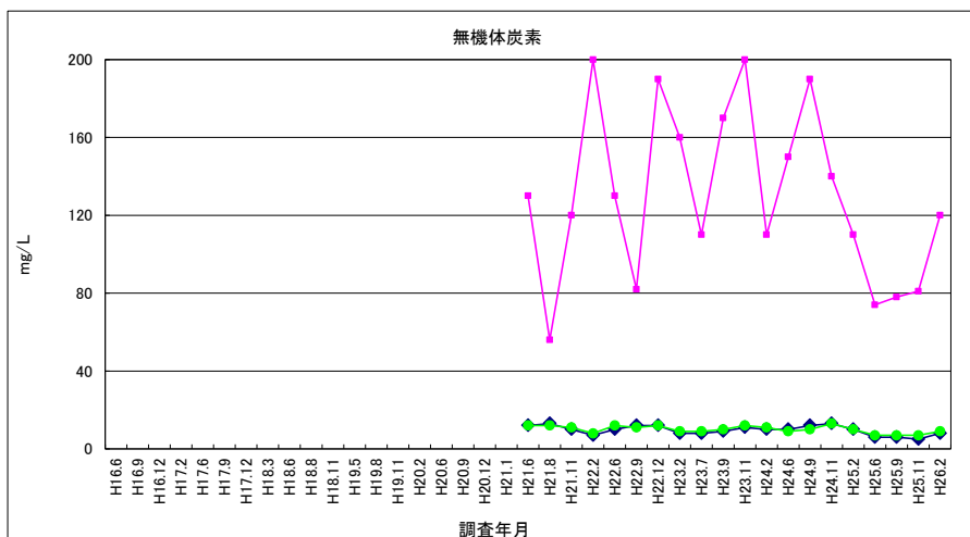
図 3-42 無機体炭素 (放流水・河川水)
