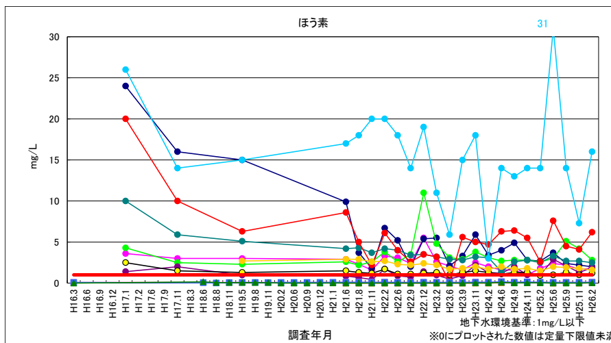
図 4-30 ほう素 (浸透水・地下水)
