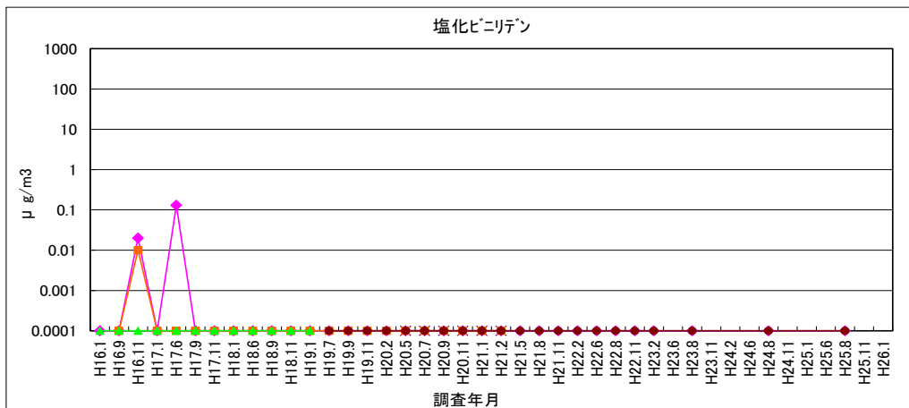
図 1-30 塩化ビニリデン
