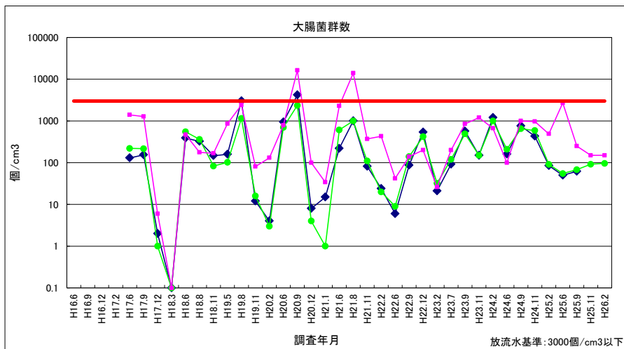
図 3-40 大腸菌群数 (放流水・河川水) ※0.1にプロットされた数値は0個/cm 3 を表す
