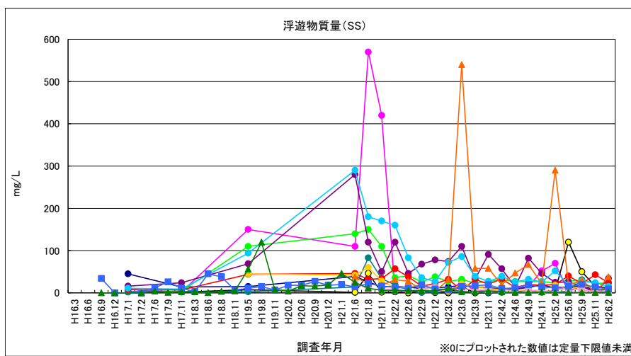
図 4-29 浮遊物質 (SS) (浸透水・地下水)
