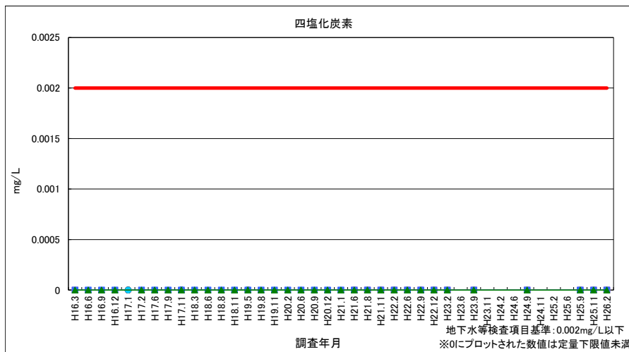
図 4-12 四塩化炭素 (浸透水・地下水)
