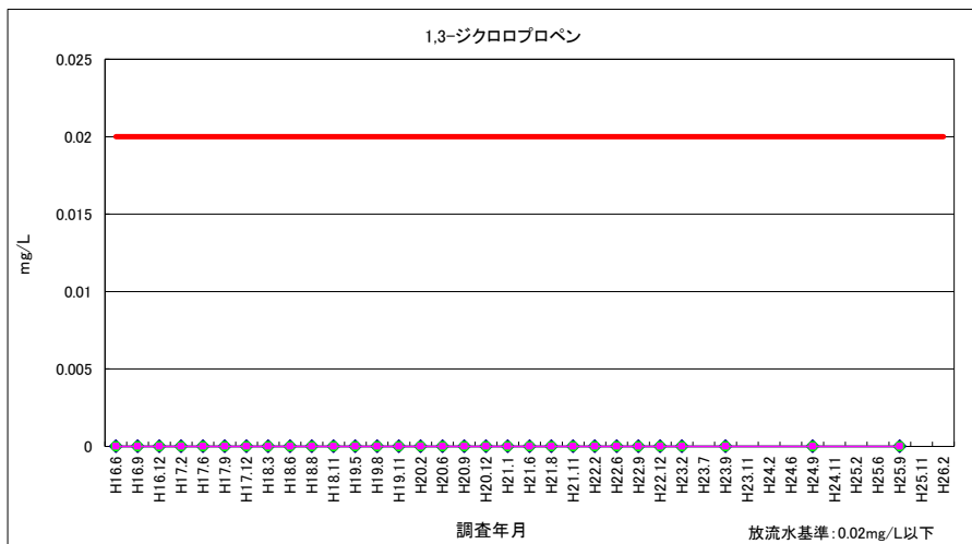
図 3-19 1,3-ジクロロプロペン (放流水・河川水)
