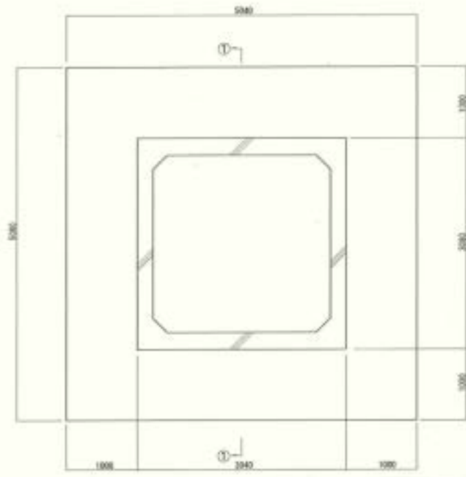
遊水壁構造図 5=1:25
