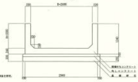
排水路構造図 5=1:25
