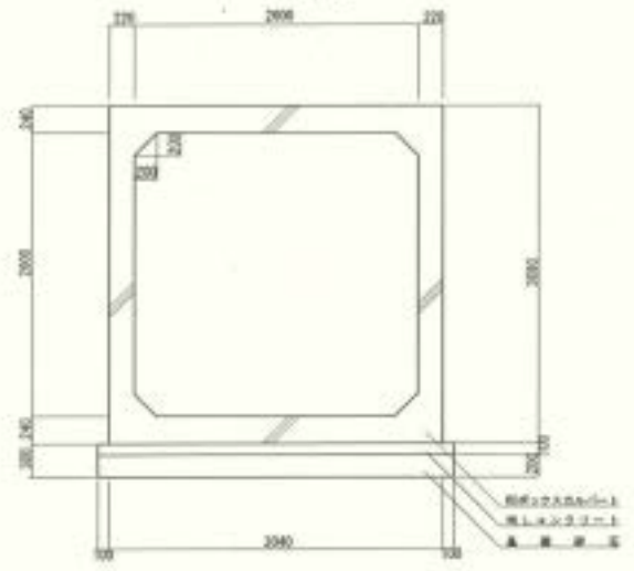
遊水壁構造図 5=1:25
