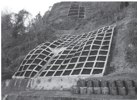
工事完成した法面
