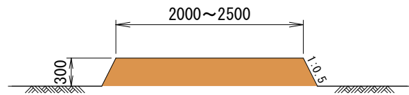
畦畔の広幅化
