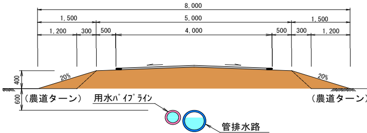
排水路の管路化
