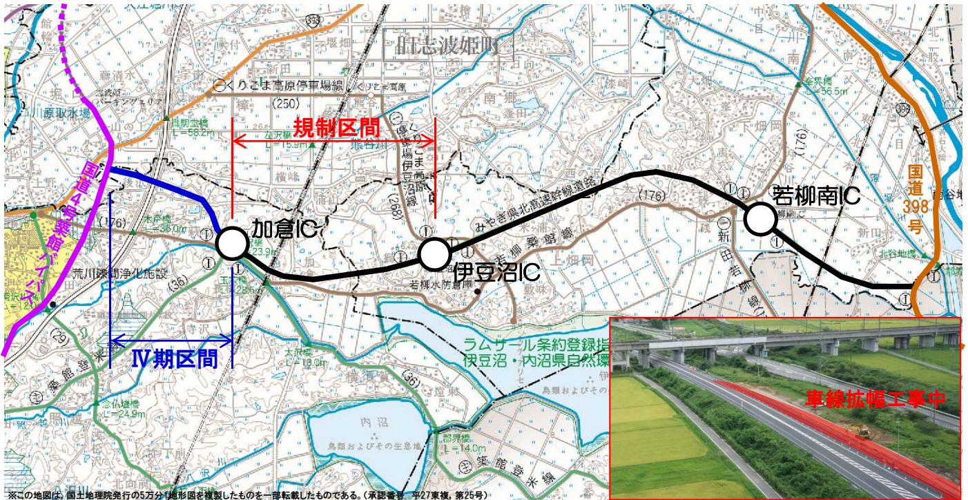
加倉IC付近の施工状況(伊豆沼IC方向を望む)
