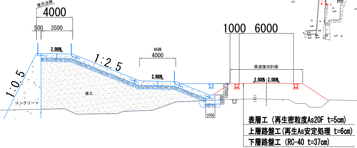
標準断面図
