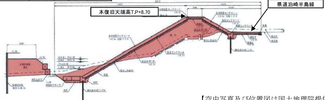
長須賀海岸災害復旧事業代表断面
