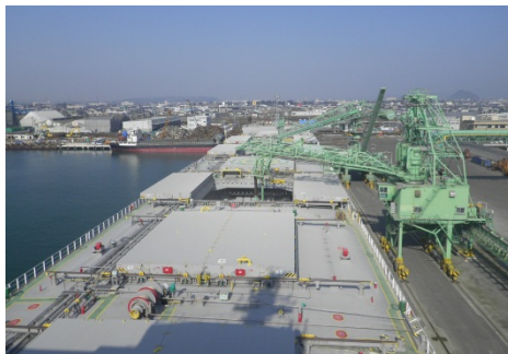
【ニューマチックアンローダーによる荷役状況】
