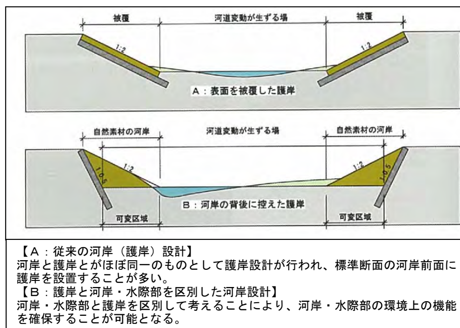
図 2-32 多自然川づくりの断面設定の考え方
