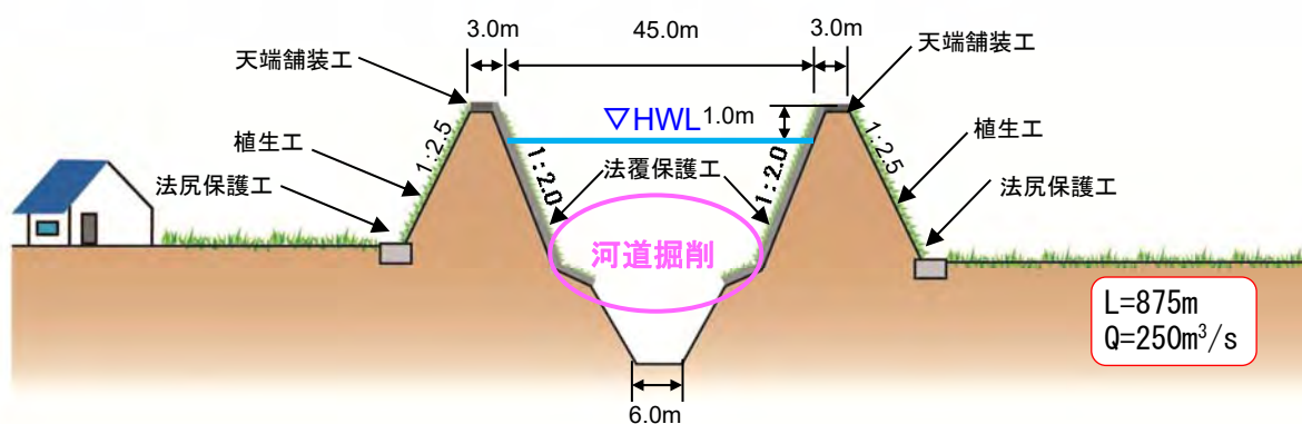
図 2-8 五福谷川下流の現況河道イメージ
