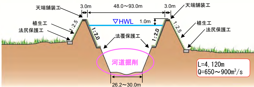
図 2-4 内川中～下流部の現況河道イメージ
