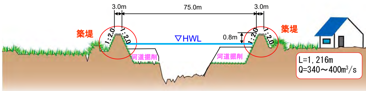
図 2-24 雫子尾川上流部（延伸区間）の現況河道イメージ
