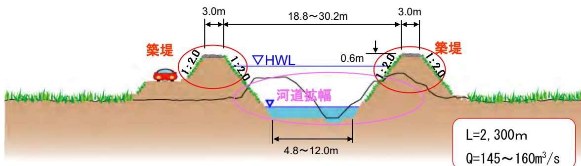
図 2-30 小田川中・上流部の現況河道イメージ
