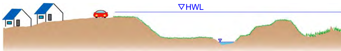
図 2-28 小田川下流部の現況河道イメージ
