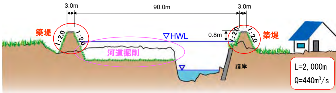
図 2-22 雫子尾川上流部の現況河道イメージ
