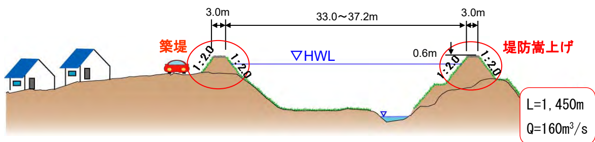
図 2-28 小田川下流部の現況河道イメージ
