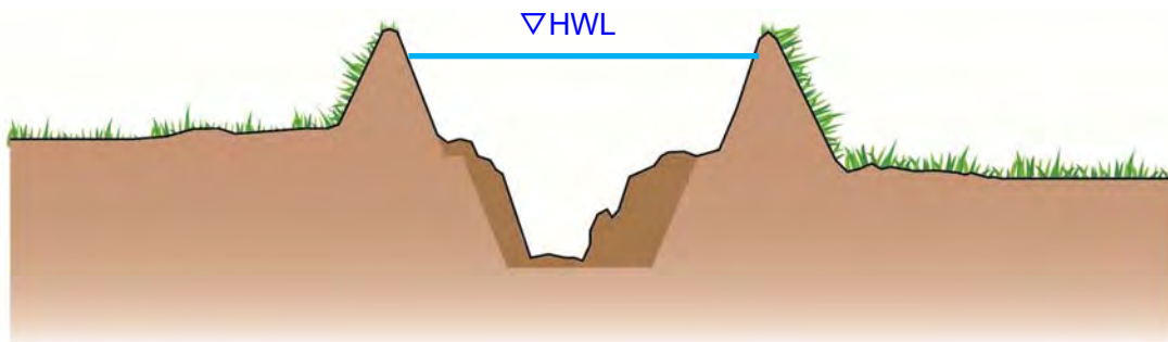
図 2-4 内川中～下流部の現況河道イメージ
