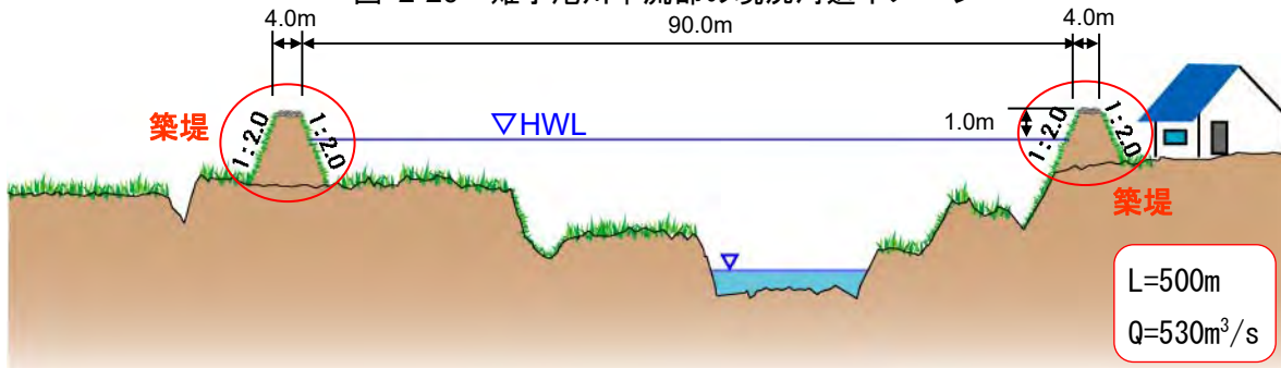
図 2-20 雫子尾川中流部の現況河道イメージ
