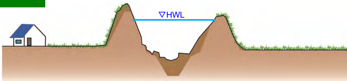
図 2-8 五福谷川下流の現況河道イメージ
