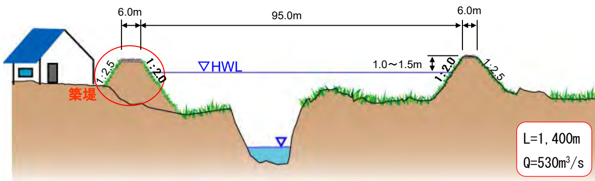
図 2-18 雫子尾川下流部の現況河道イメージ
