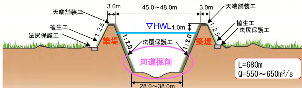
図 2-7 内川上流部の改修イメージ
