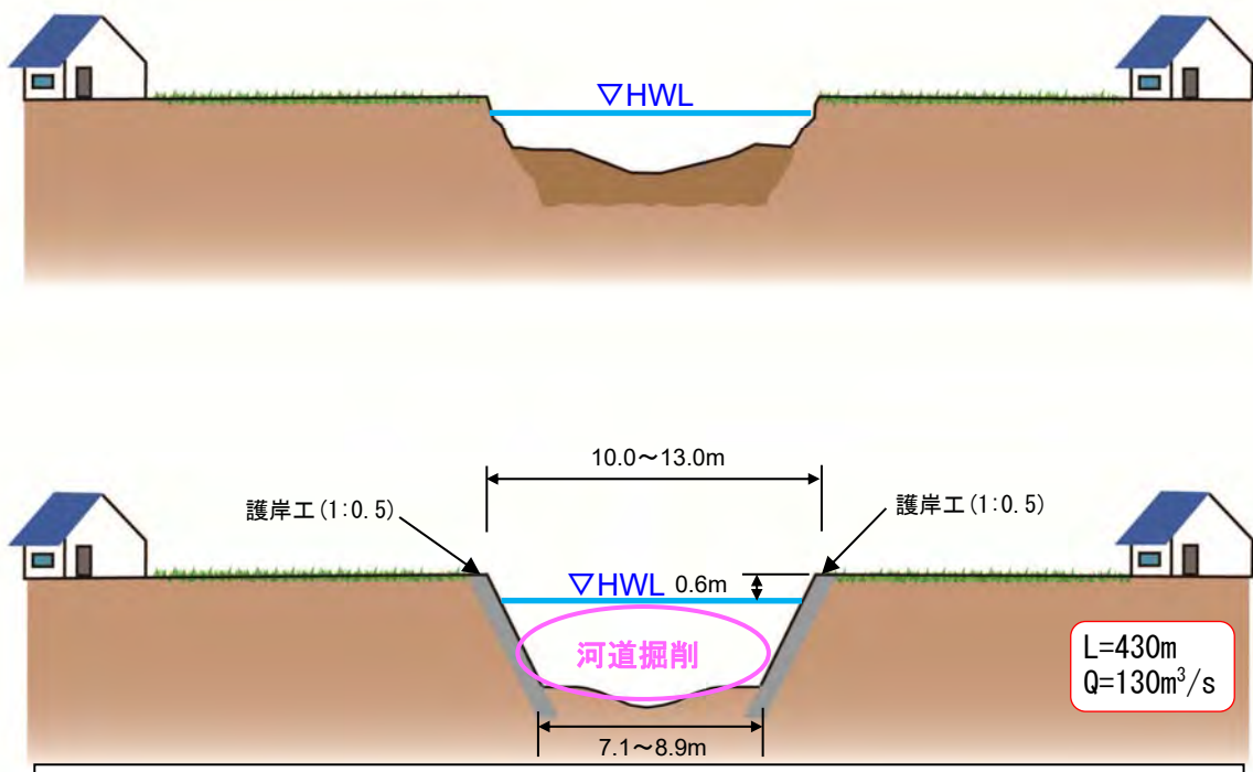
図 2-15 新川上流の改修イメージ
