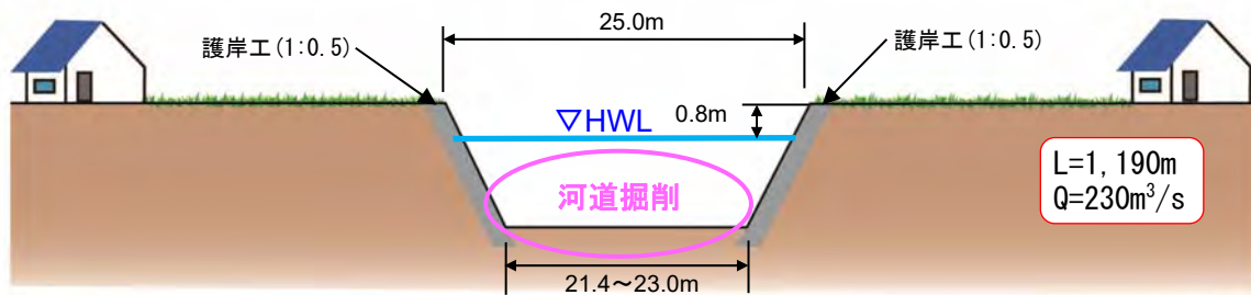
図 2-11 五福谷川上流の改修イメージ
