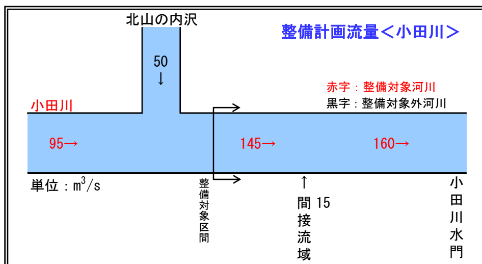
図 2-27 流量配分図
