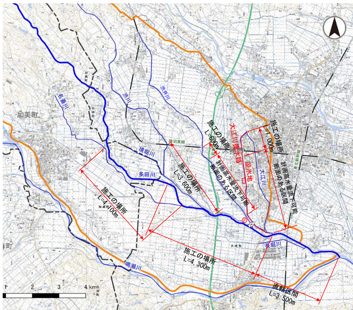
図 19 整備計画位置図
