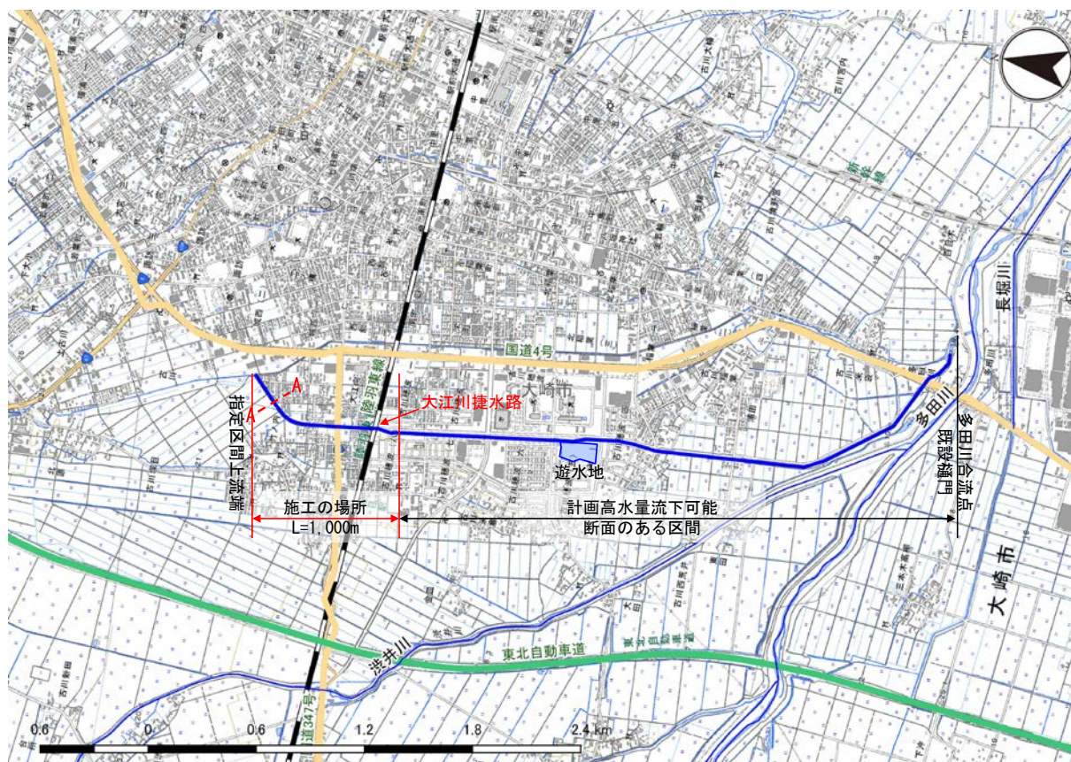
図 28 整備実施区間位置図
