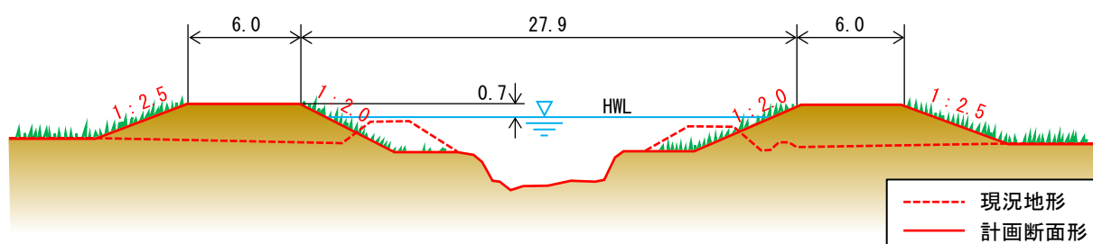
図 27 横断面図(多田川合流点から 2,000m)
