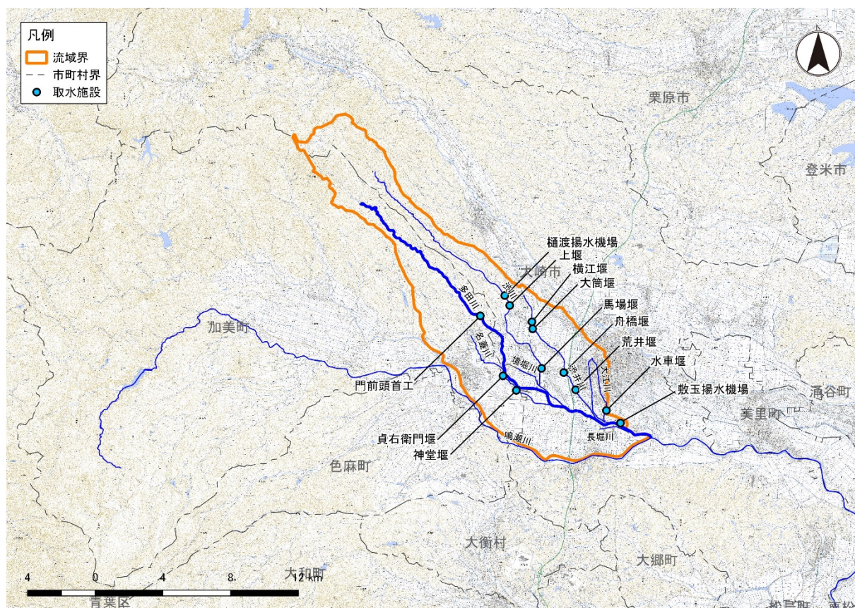
図 15 多田川流域の取水施設
