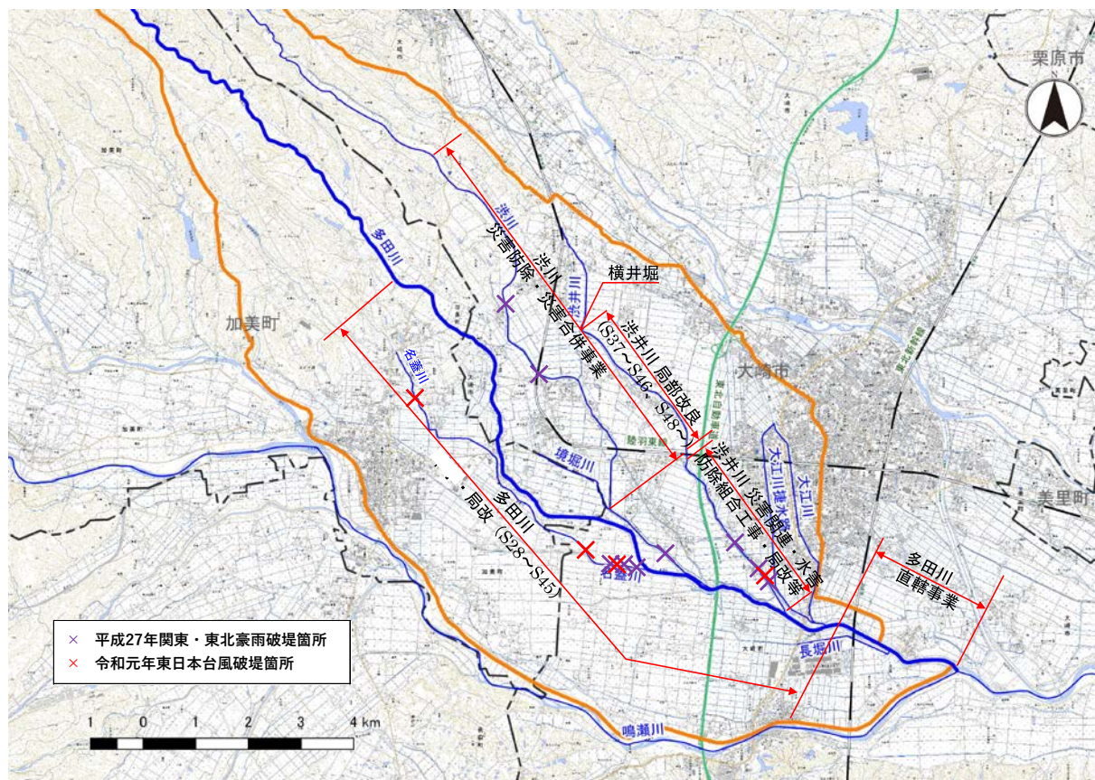
図 13 多田川流域の改修履歴
