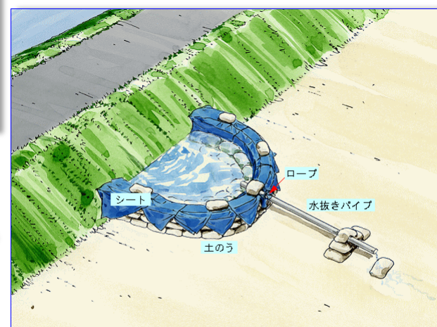
月の輪工法 完成図
