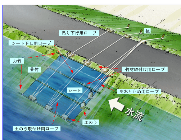
シート張り工法 完成図
