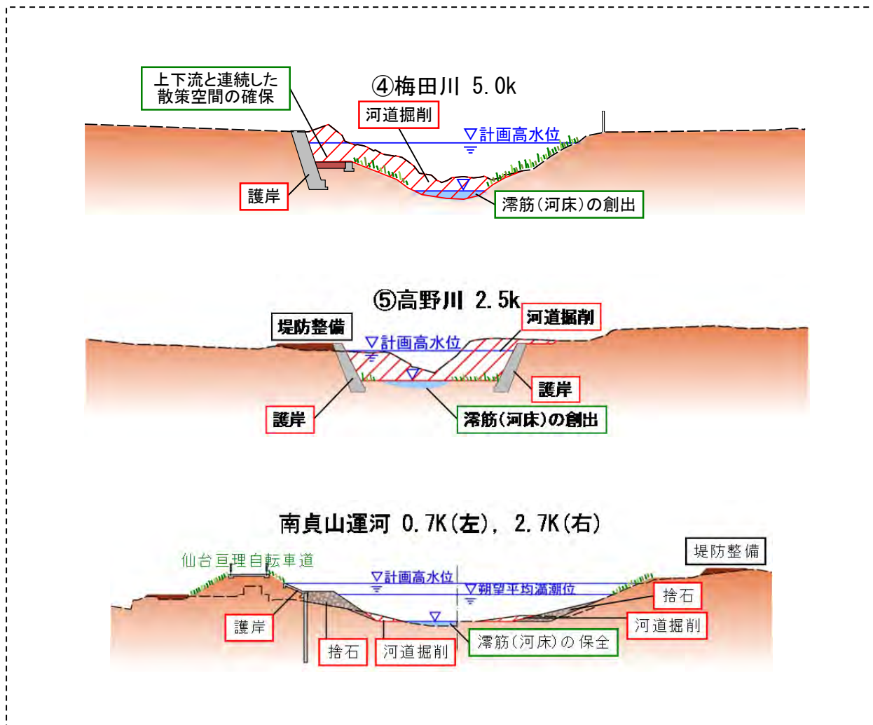
図 2.2 河川改修のイメージ図(2)
