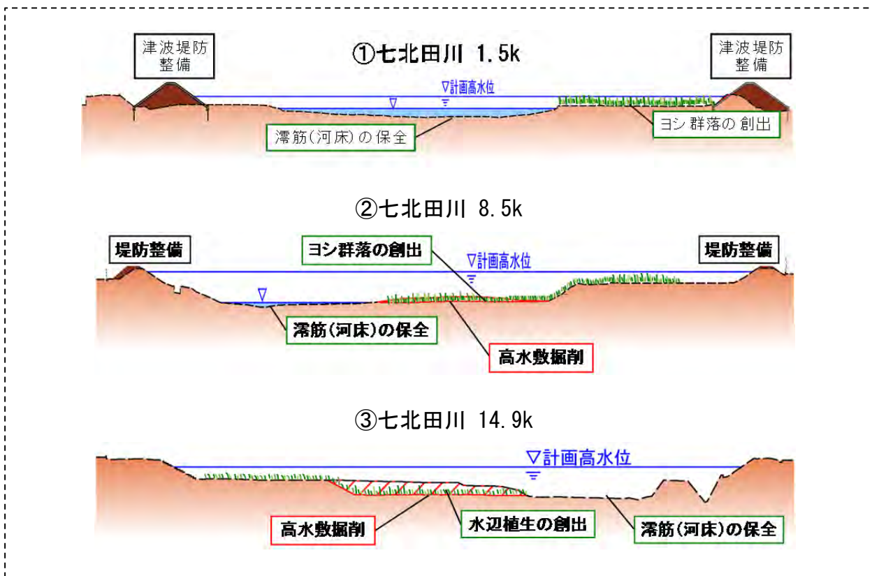
図 2.2 河川改修のイメージ図(1)
