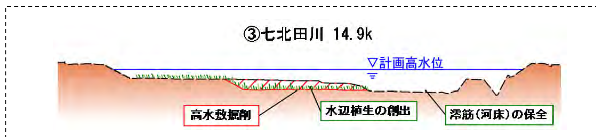
図 2.4 河道掘削横断のイメージ図
