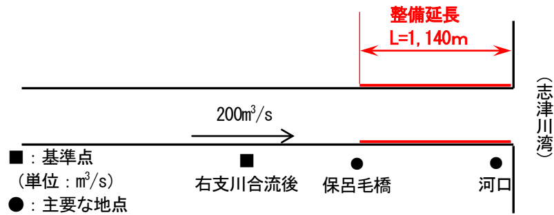
水尻川計画高水流量図
