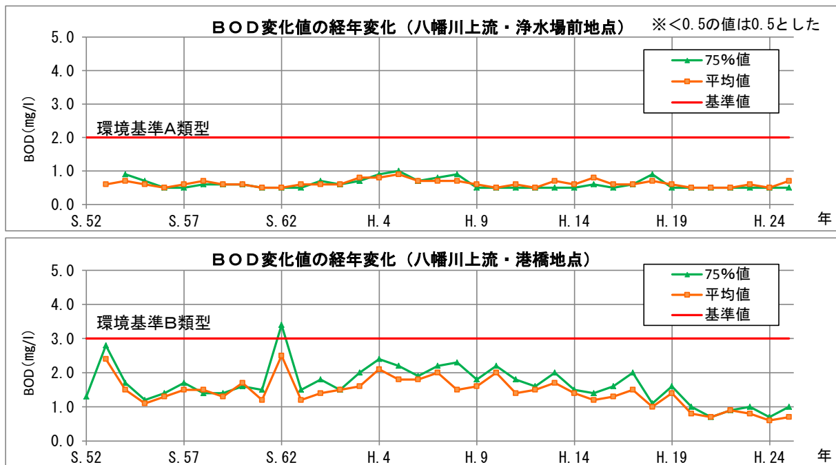
図 1-26 BOD 変遷図【八幡川：浄水場前、港橋】
