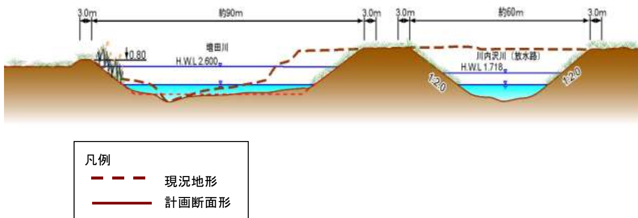
図2-3 増田川代表横断面図 (A 地点)
