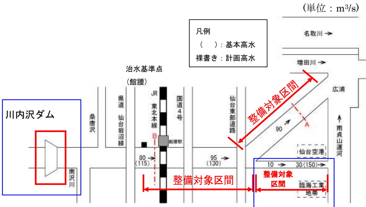
図2-4 川内沢川計画高水流量配分図
