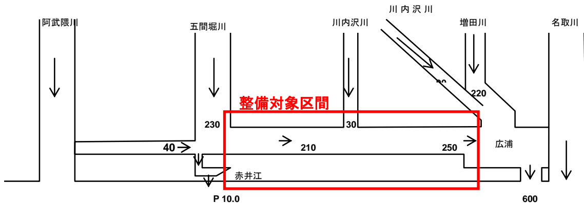
図 2-7 南貞山運河計画流量配分図
