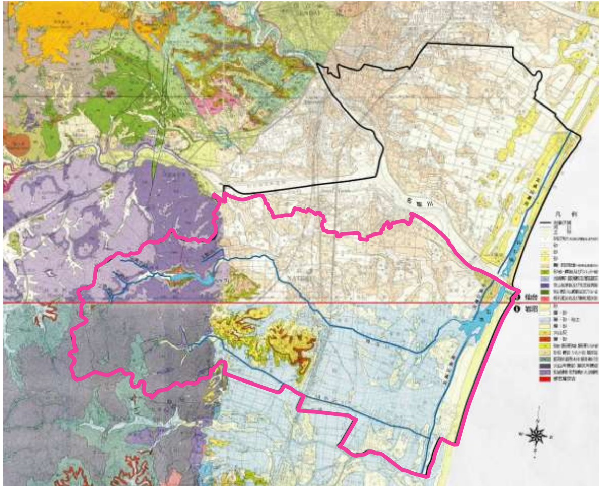
図1-3 表層地質図
