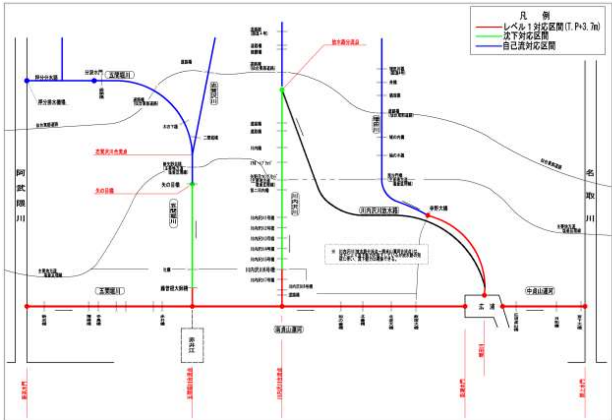
図 2-10 明治三陸地震規模津波での波遡上高対応の堤防整備範囲
