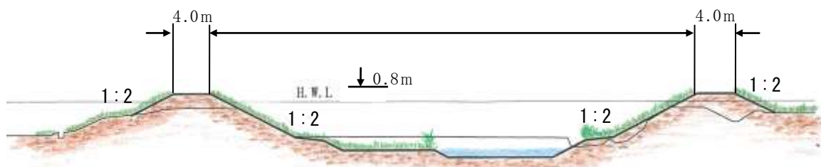
横断図 (南沢川水門から 2.8km 上流付近)
