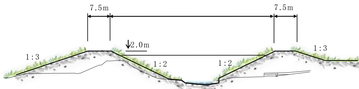
横断面図（北上川合流点から 0.2km 上流付近）
