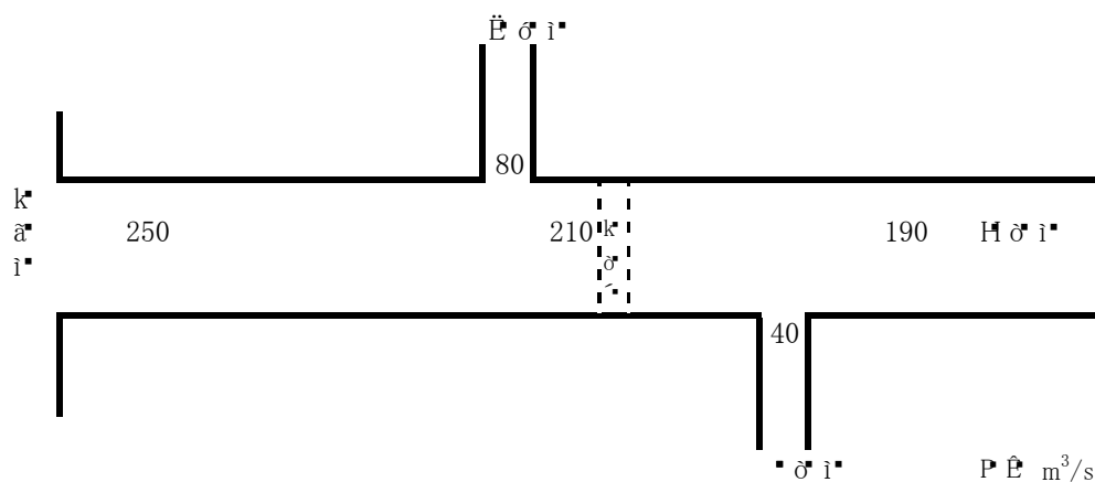
整備計画流量配分（羽沢川）
