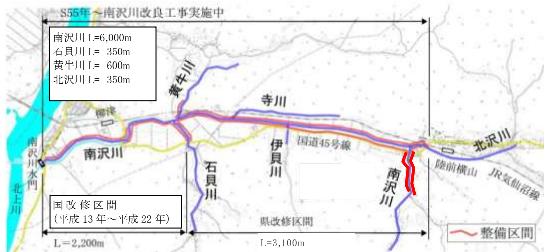
整備計画位置
