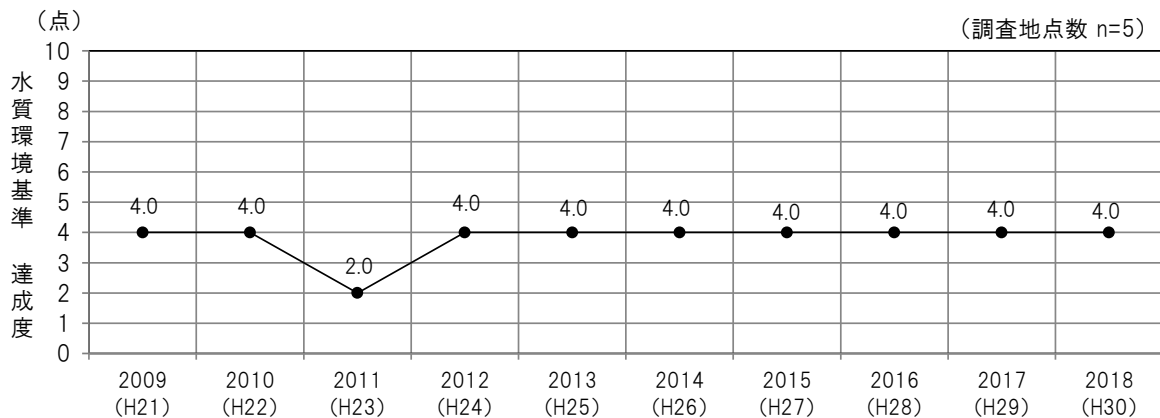
図 3.14 水質環境基準の達成度の経年変化図(湖沼 全 りん 燐)
