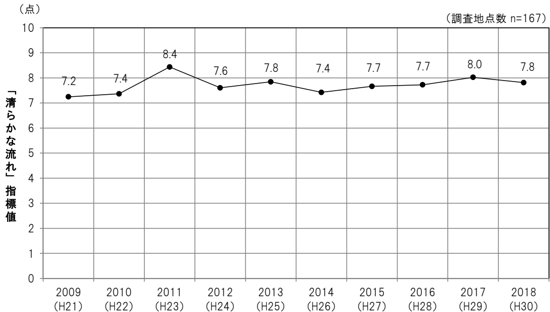
図 3.11 「清らかな流れ」指標値の経年変化図
