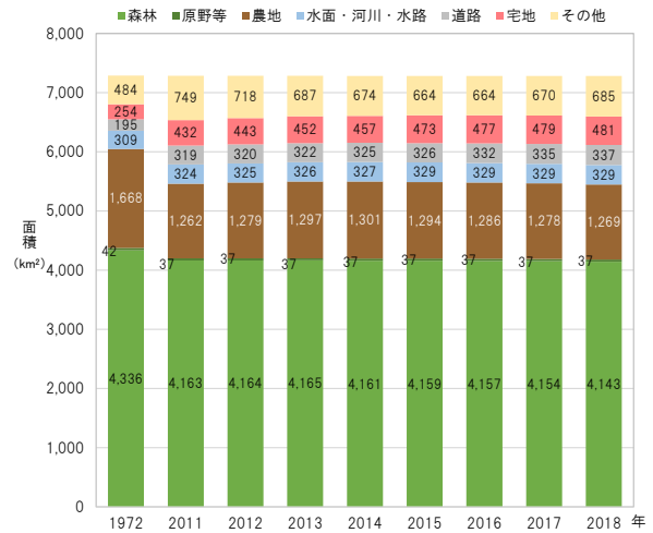
図 3.6 土地利用現況の推移
