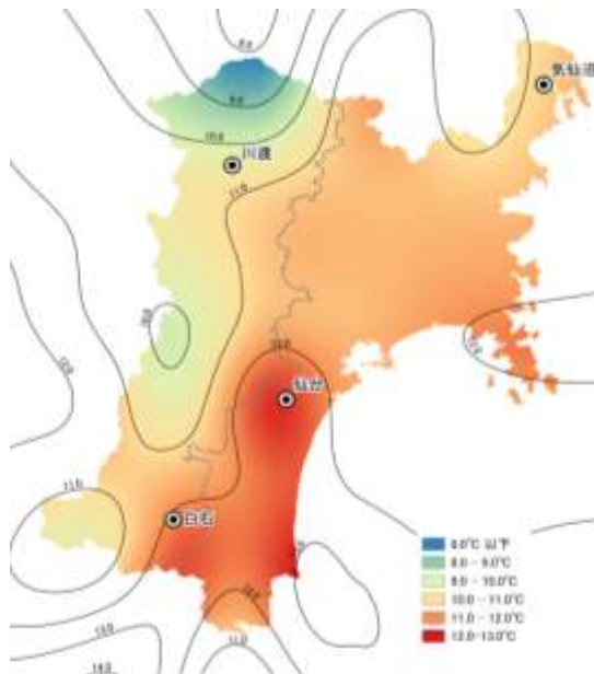
図 3.4 等温線図
