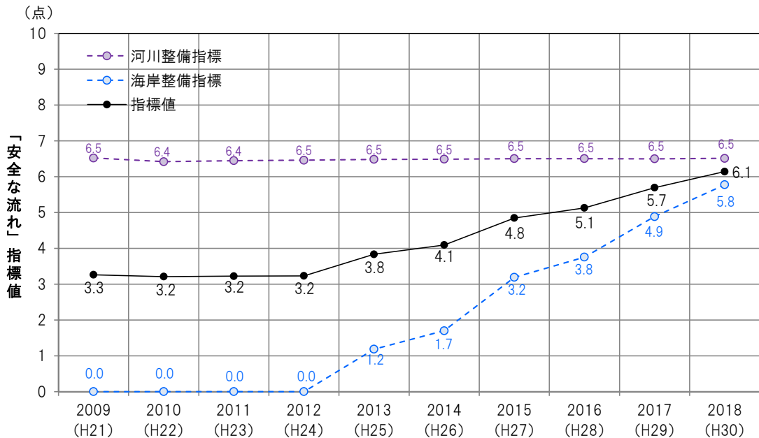
図 3.19 「安全な流れ」指標値の経年変化図
