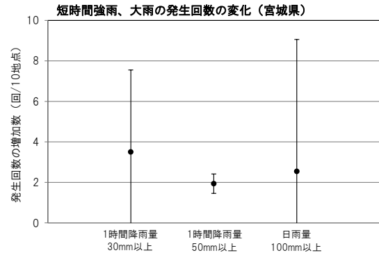
図 3.10 短時間豪雨、大雨の発生回数の変化
