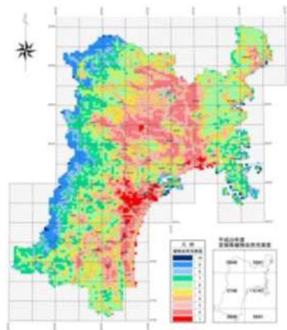
図 5.10 植物自然充実度
