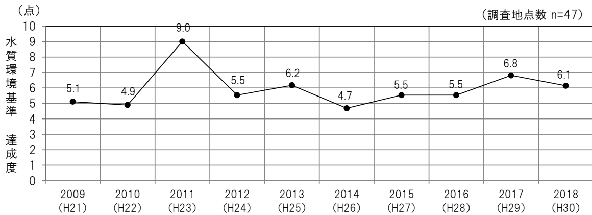
図 3.15 水質環境基準の達成度の経年変化図(海域 COD)
