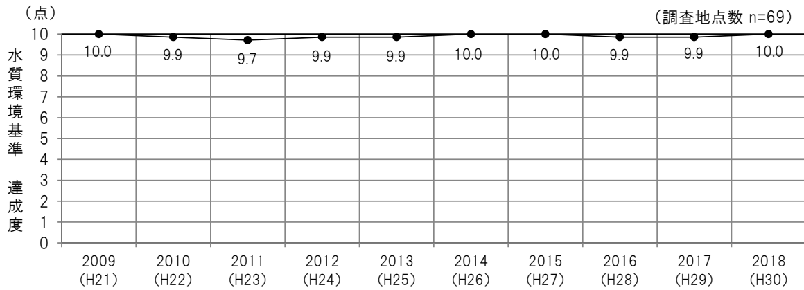
図 3.12 水質環境基準の達成度の経年変化図(河川 BOD)
