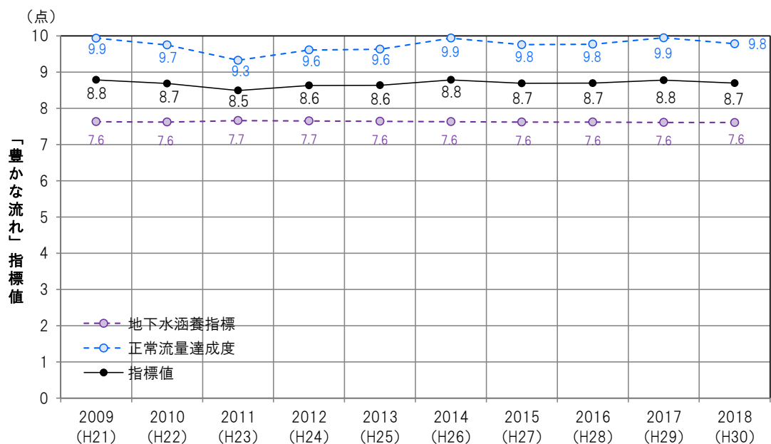
図 3.18 「豊かな流れ」指標値の経年変化図
