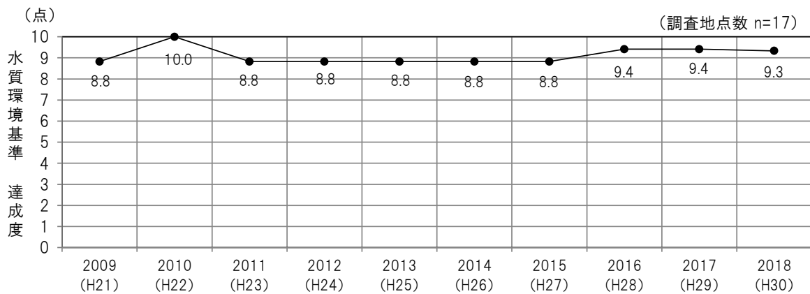
図 3.16 水質環境基準の達成度の経年変化図(海域 全窒素)
