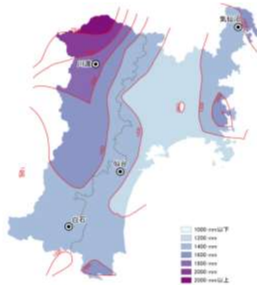
図 3.5 等雨量線図
