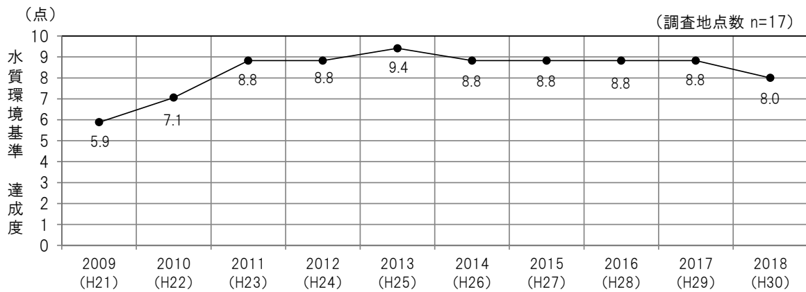
図 3.17 水質環境基準の達成度の経年変化図(海域 全リン)
