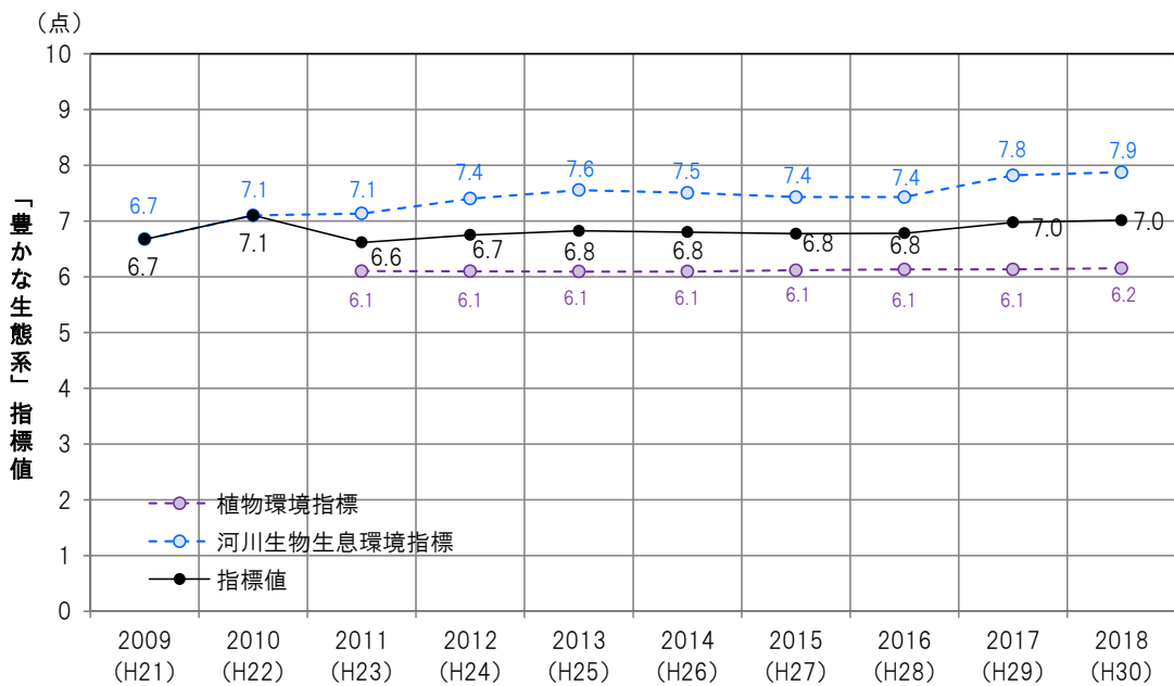
図 3.20 「豊かな生態系」指標値の経年変化図
