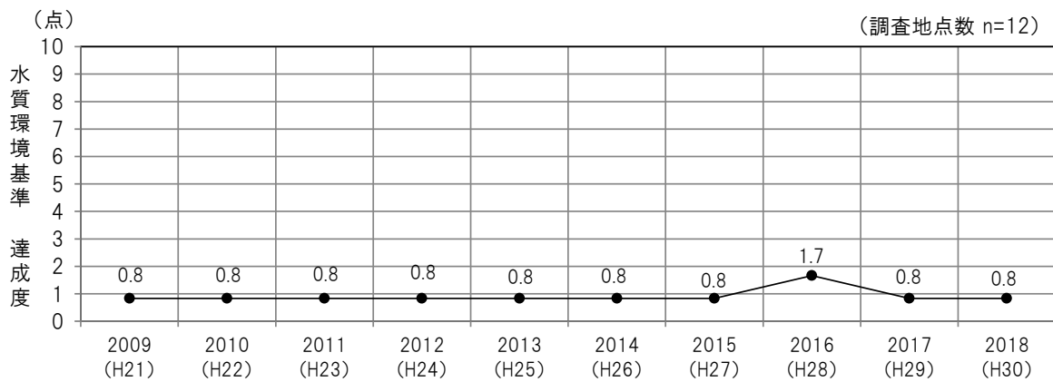
図 3.13 水質環境基準の達成度の経年変化図(湖沼 COD)
