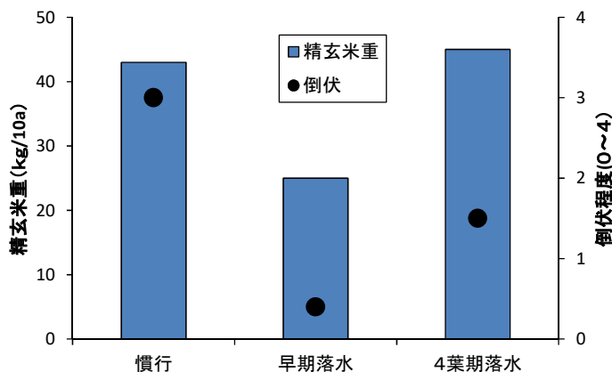
収量と倒伏 (H26年: 古川農試)
