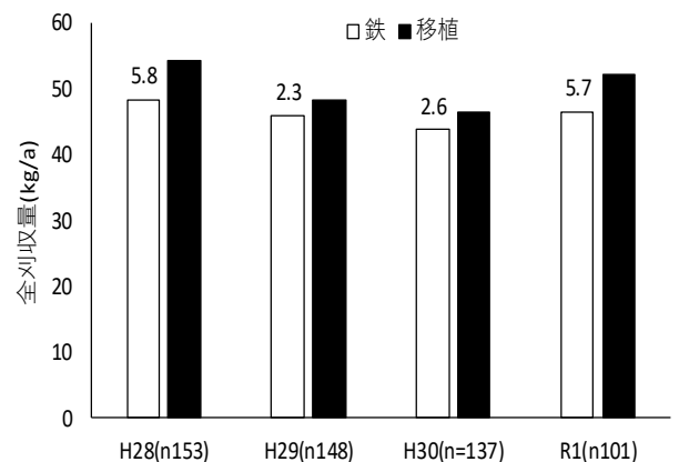
鉄コーティングと移植の収量差 (H28～R1年:(株)五十嵐商会)
