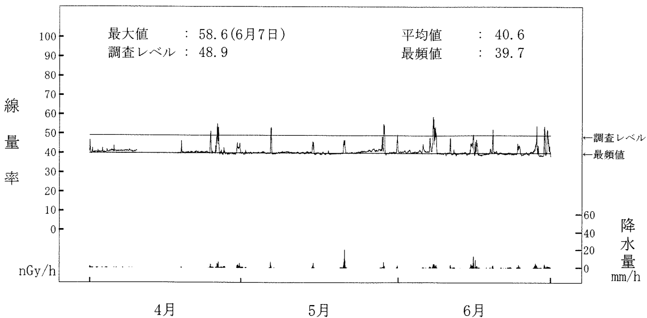
図-2-9 空間ガンマ線量率監視結果 (寺間局)
