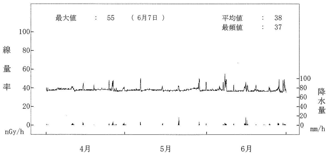
空間ガンマ線量率監視結果(MP-2)
