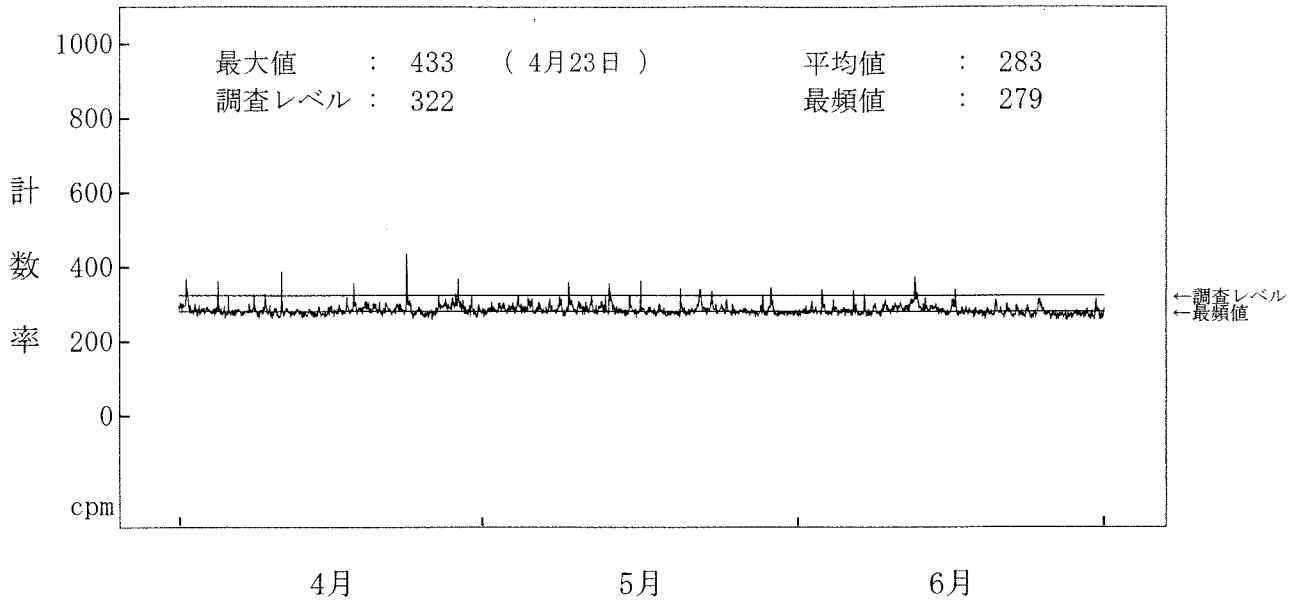
図-2-12 海水(放水)中の全ガンマ線計数率監視結果(1号機放水口モニター(A))
