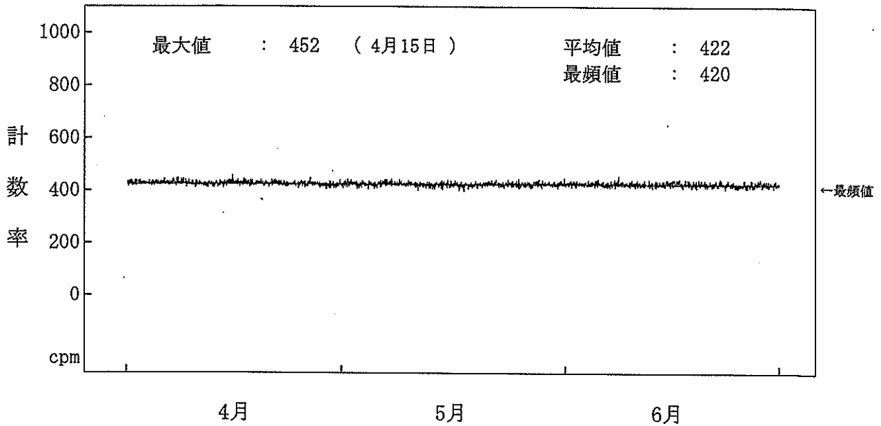
図-2-14 海水(放水)中の全ガンマ線計数率監視結果(2号機放水口モニター) (注) 4月24日、5月22日及び6月12日～13日の欠測は、定期点検によるものである。
