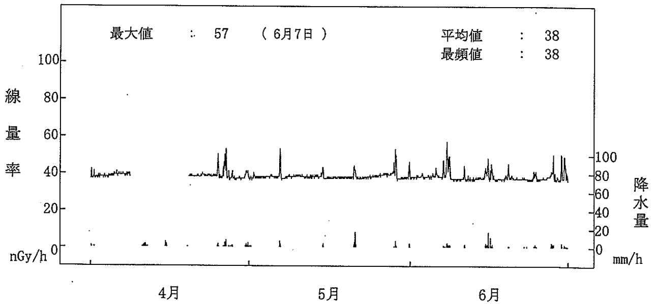
空間ガンマ線量率監視結果(MP-5)
