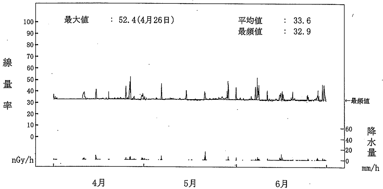
図-2-10 空間ガンマ線量率監視結果(江島局) (注) 4月2日~4月10日の欠測は、非常用発電機設置工事によるものである。
