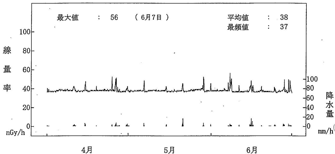
空間ガンマ線量率監視結果(MP-3)
