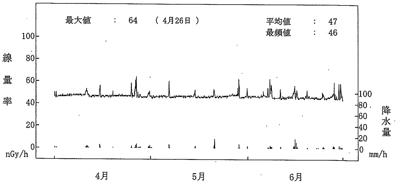
空間ガンマ線量率監視結果(MP-6)
