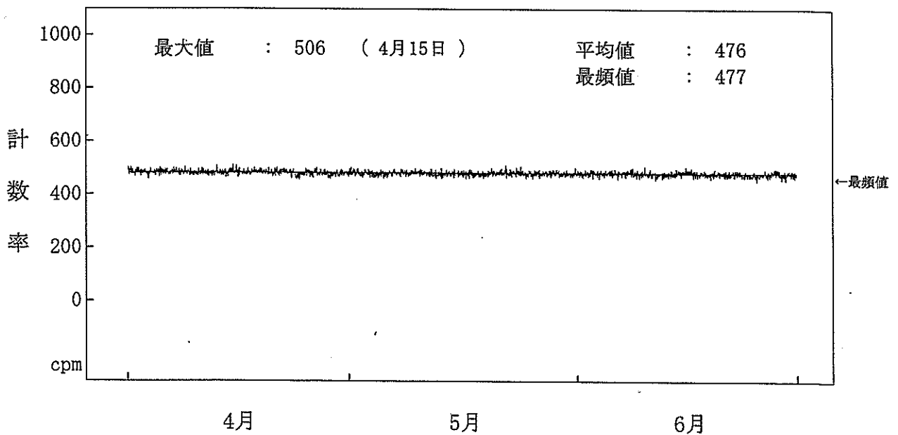
図-2-15 海水(放水)中の全ガンマ線計数率監視結果(3号機放水口モニター) (注) 4月23日、5月15日及び6月11日～12日の欠測は、定期点検によるものである。
