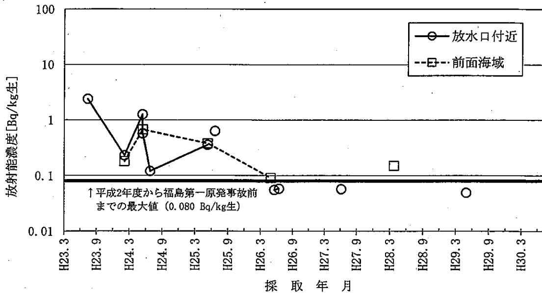
図-2-20 ワカメのCs-137濃度の推移
