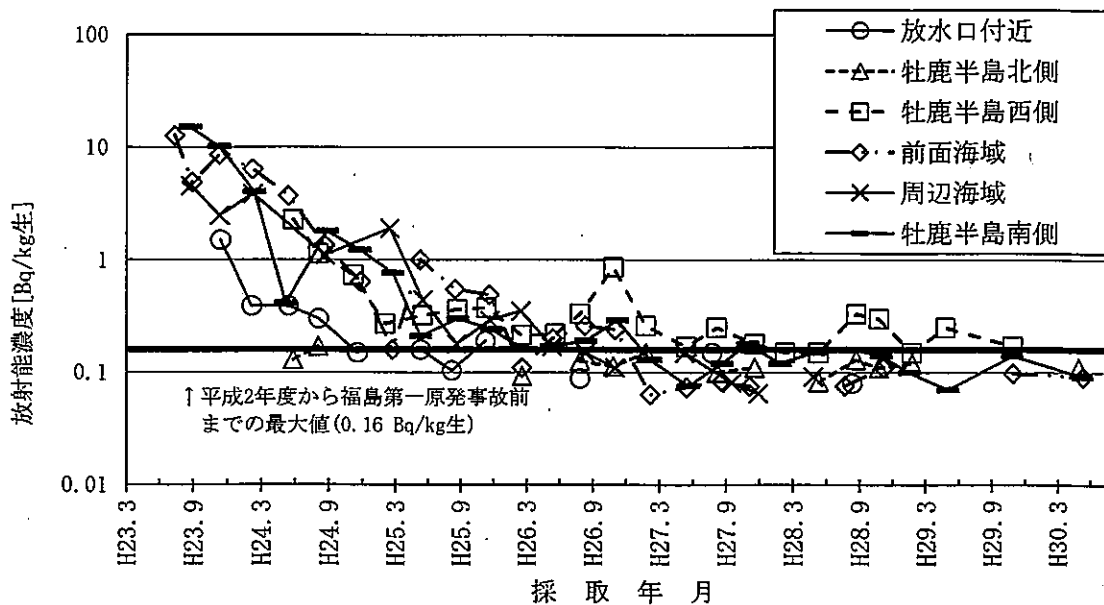
図-2-23 アラメのCs-137濃度の推移
