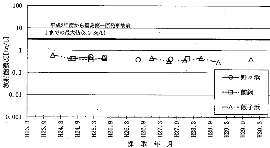
図-2-28 陸水のH-3濃度の推移
