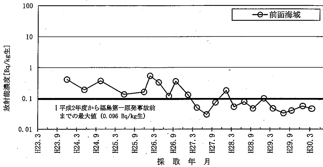
図-2-24 ムラサキガイのCs-137濃度の推移
