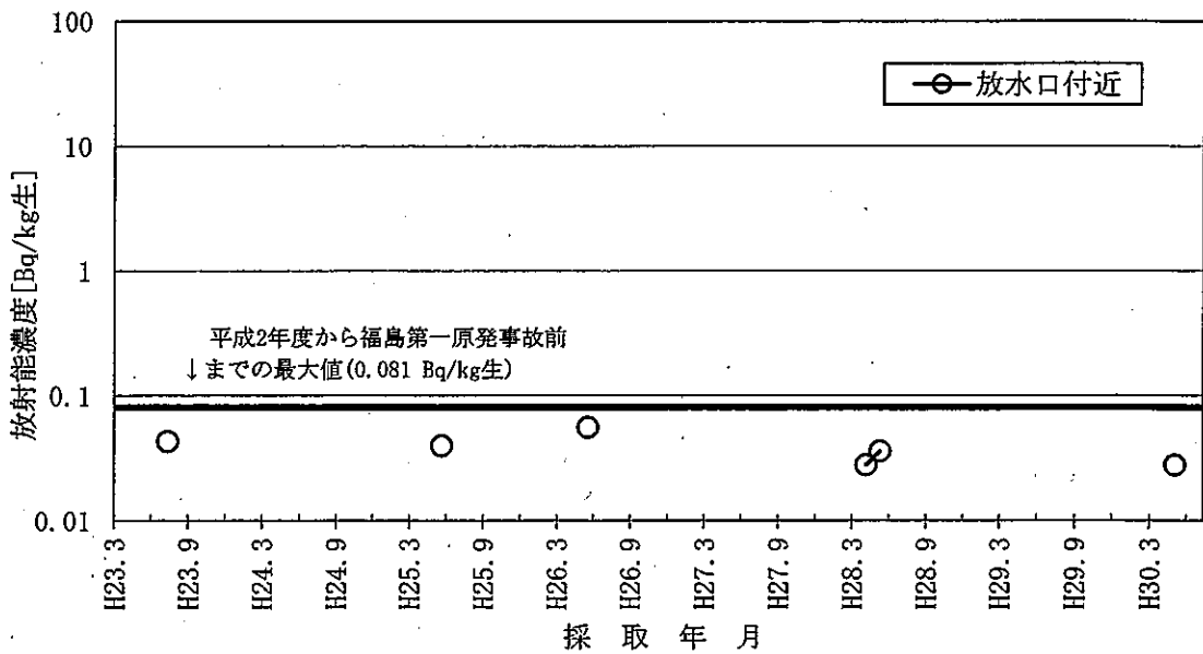
図-2-26 ワカメのSr-90濃度の推移
