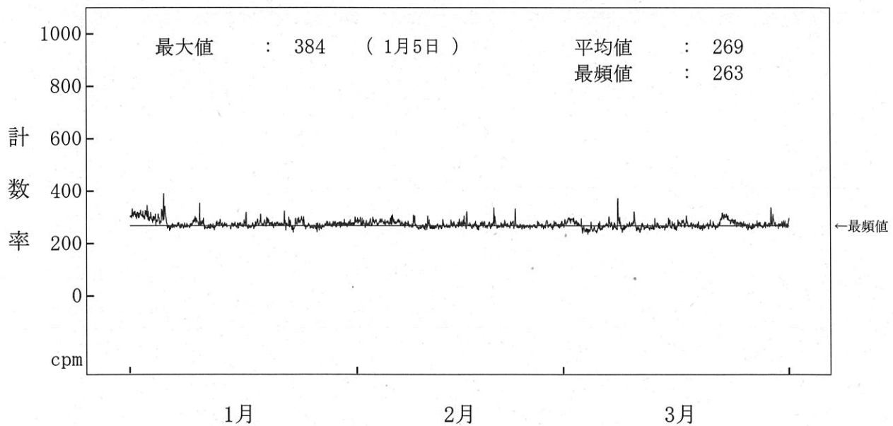
図-2-9 海水(放水)中の全ガンマ線計数率監視結果(1号機放水口モニター(B)) (注) 1月14日の欠測は、構内配電線の停電作業によるものである。
