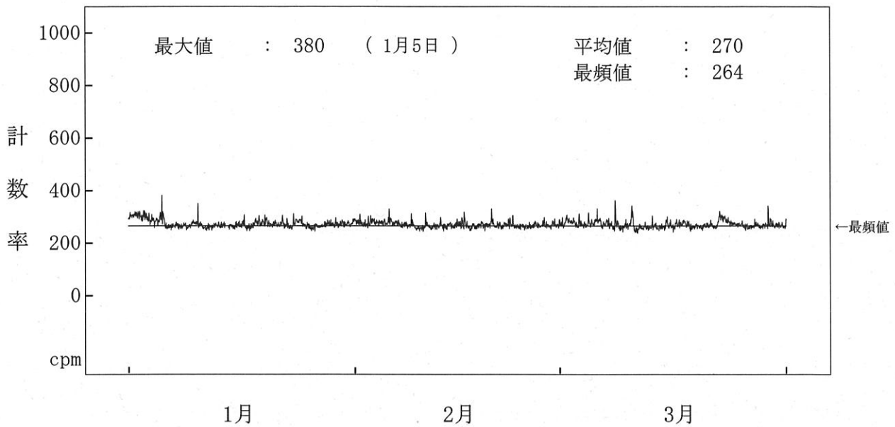
図-2-8 海水(放水)中の全ガンマ線計数率監視結果(1号機放水口モニター(A)) (注) 1月14日の欠測は、構内配電線の停電作業によるものである。
