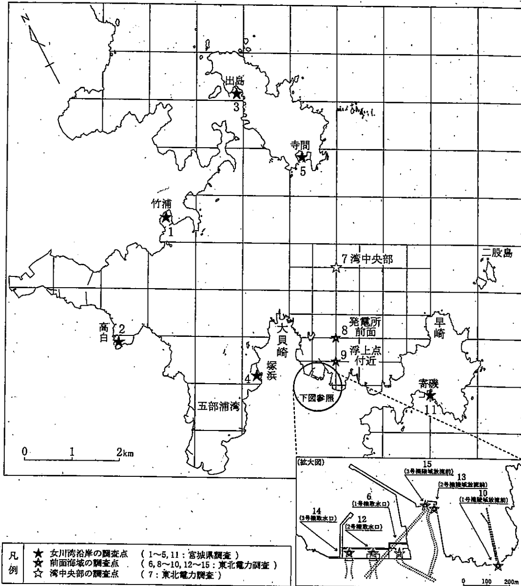
図一 7 水温調査 (モニタリング) 位置
