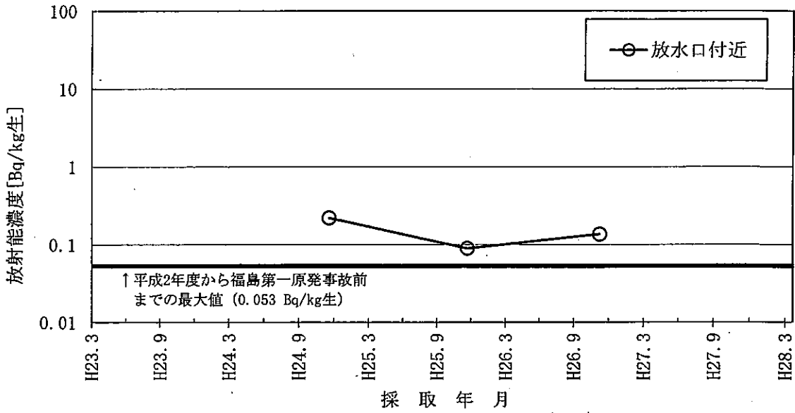
図-14 アワビのCs-137濃度の推移
