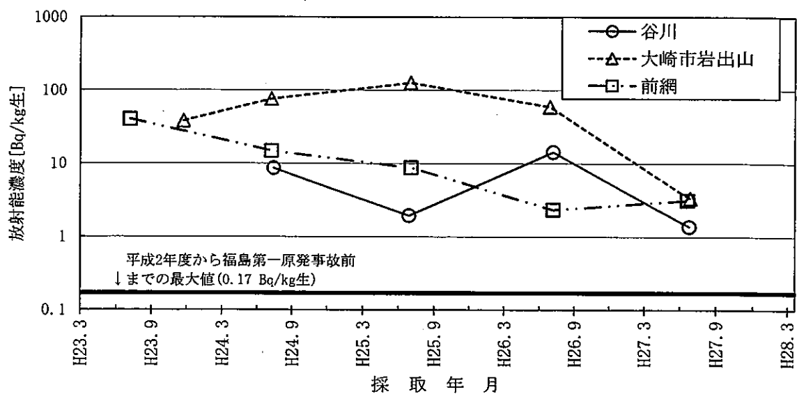
図-10 稲のCs-137濃度の推移
