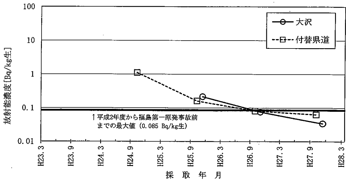
図-8 大根(葉)のCs-137濃度の推移
