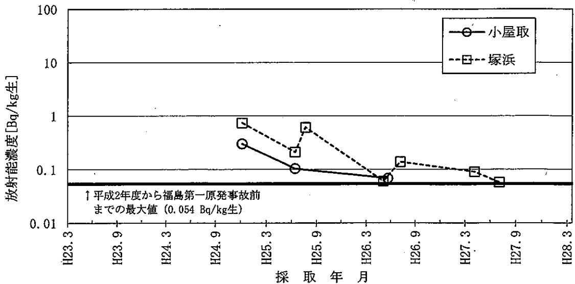
図-1 3 ホヤのCs-137濃度の推移
