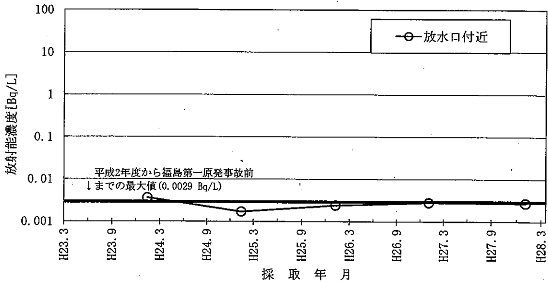
図-27 海水のSr-90濃度の推移
