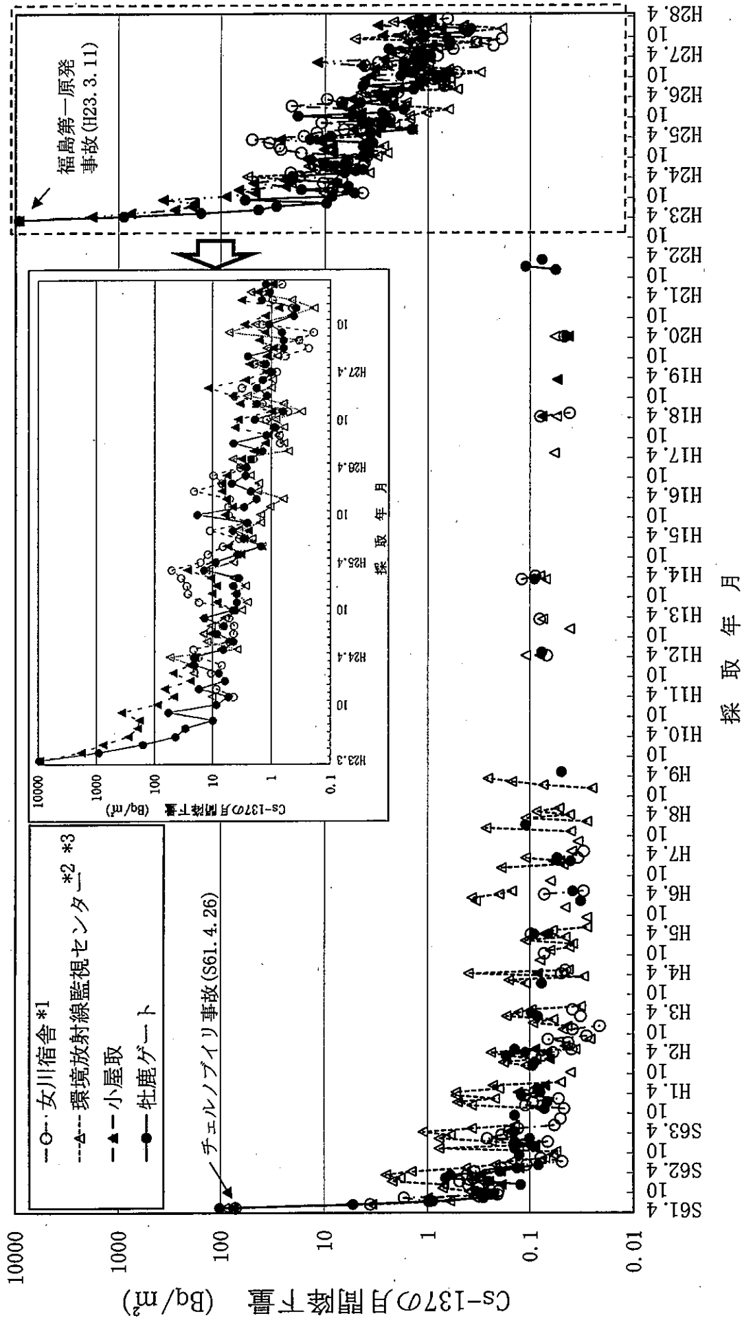
図一 2 Cs(セシウム)-137の月間降下量の推移
