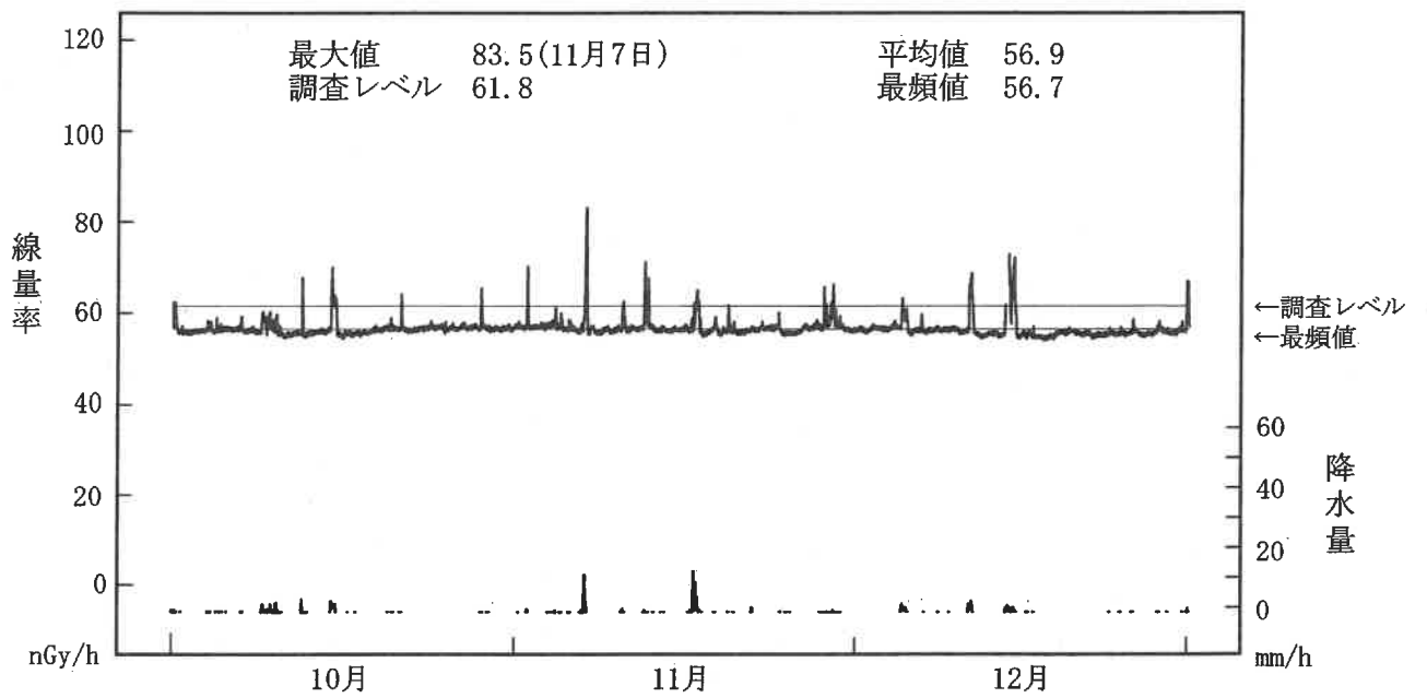
図-2-7 NaI(Tl)検出器による空間ガンマ線量率監視結果（茨浜局）
