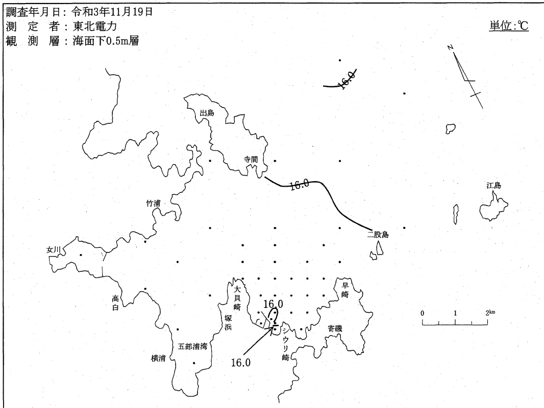
図-4-(2) 等温線
