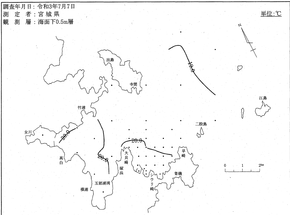
図-2-(2) 等温線
