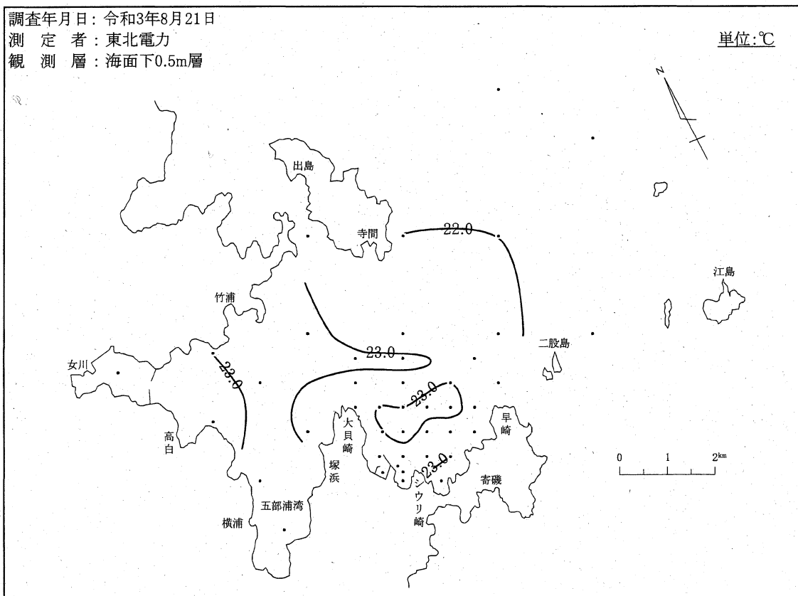
図-4-(2) 等温線
