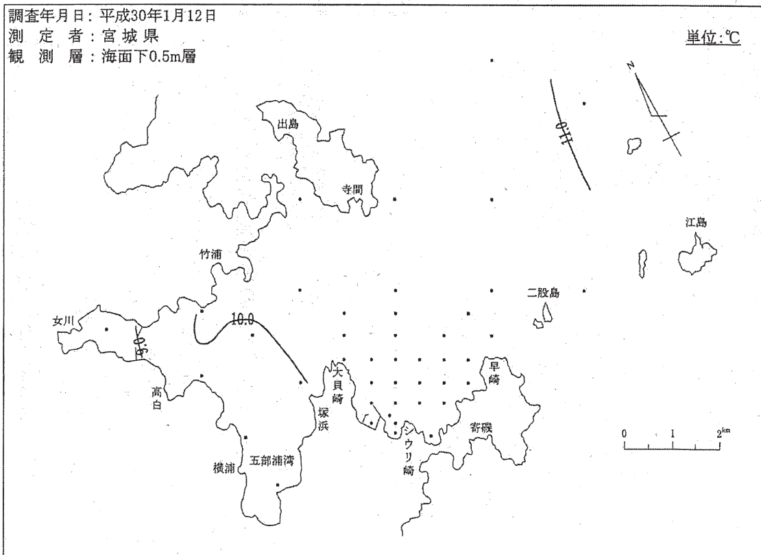
図-2-(2) 等温線
