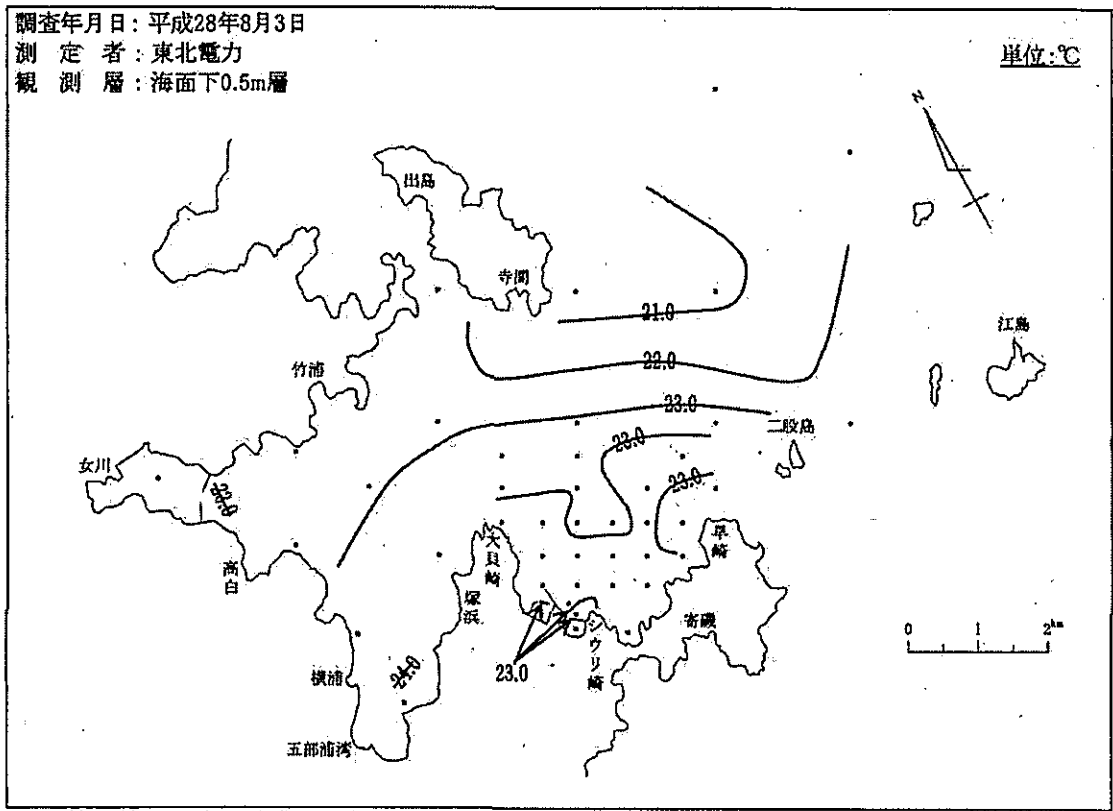
図-4-(2) 等温線
