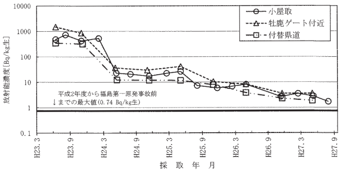
図-2-17 松葉のCs-137濃度の推移
