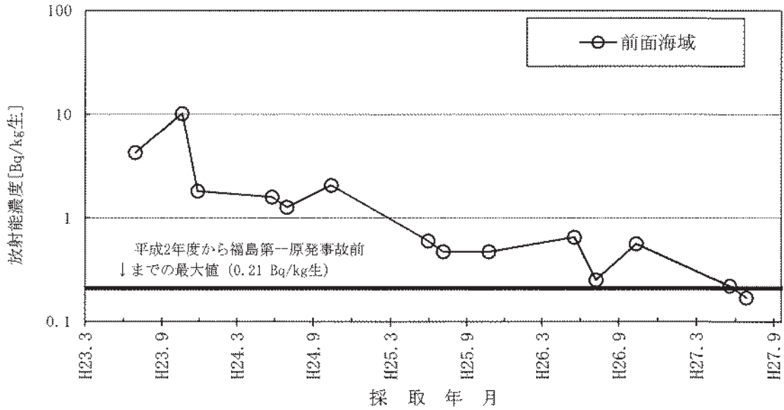
図-2-18 アイナメのCs-137濃度の推移
