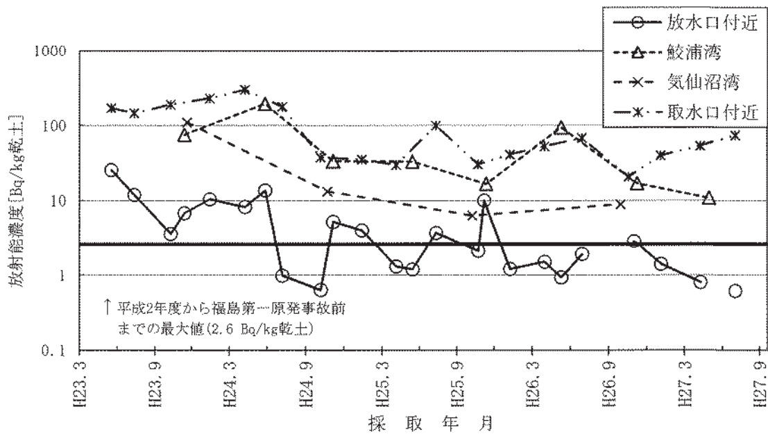
図-2-22 海底土のCs-137濃度の推移
