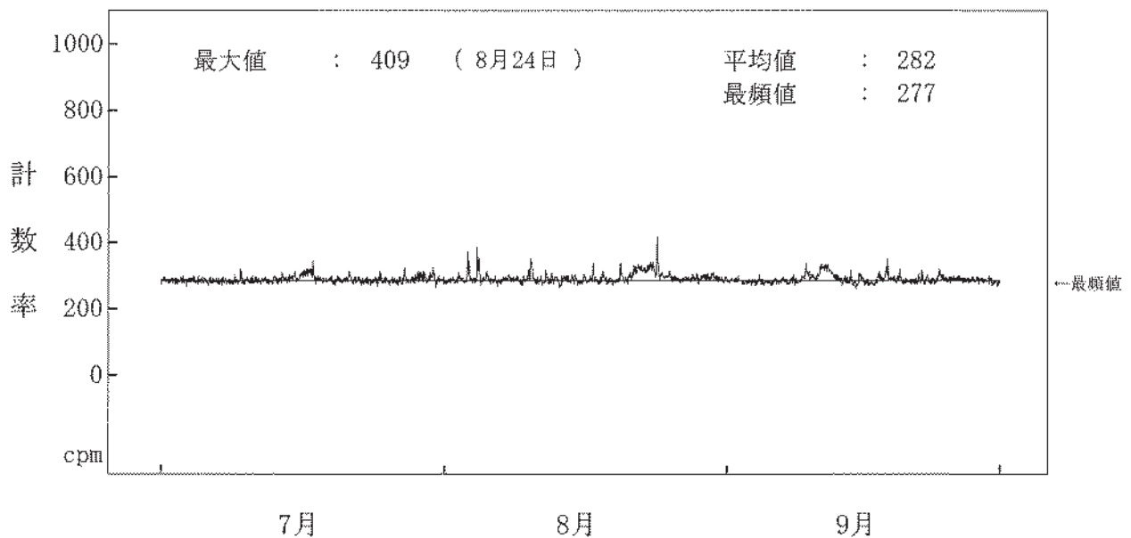
図一 2 - 8 海水(放水)中の全ガンマ線計数率監視結果(1号機放水口モニター(A))
