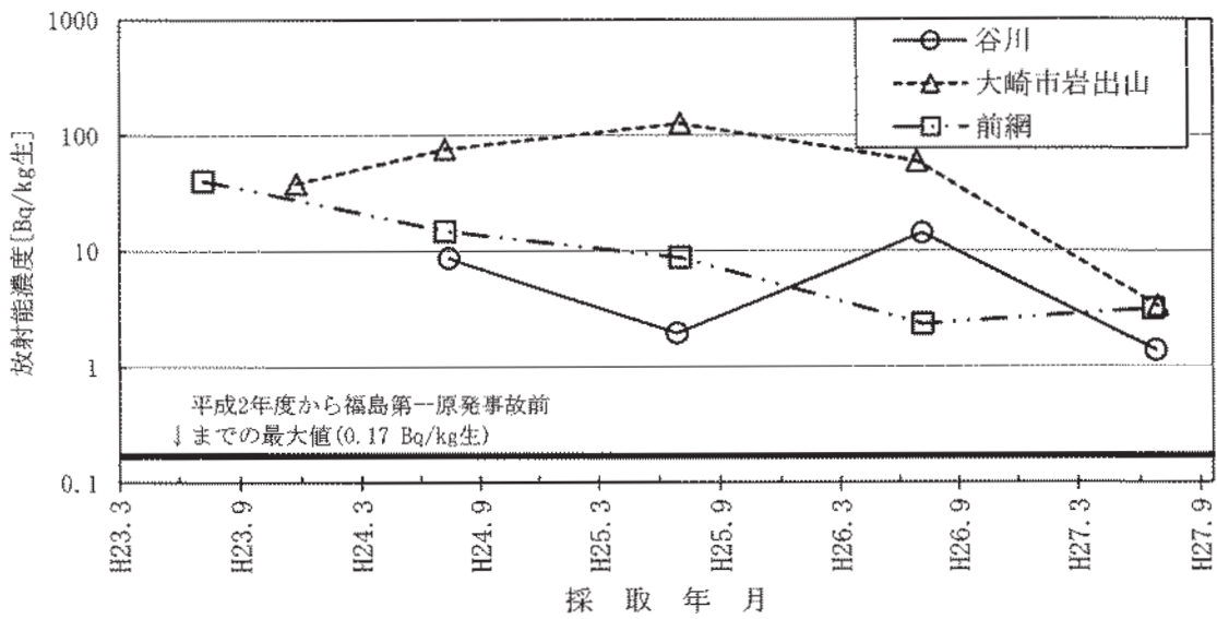
図-2-16 ヨモギのCs-137濃度の推移
