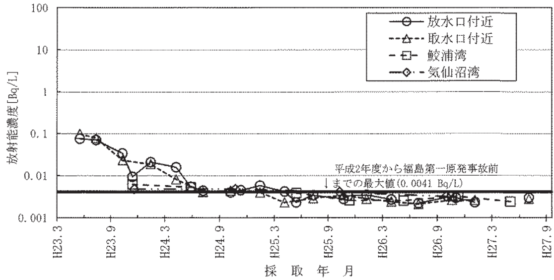
図-2-21 海水のCs-137濃度の推移
