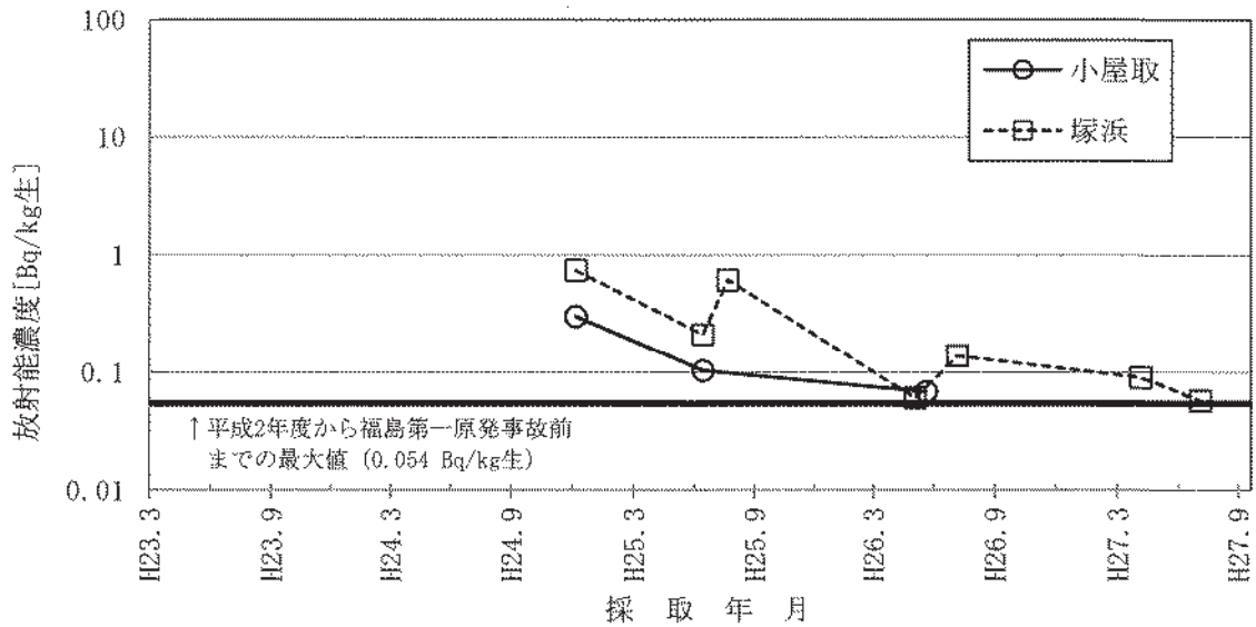
図-2-19 ホヤのCs-137濃度の推移
