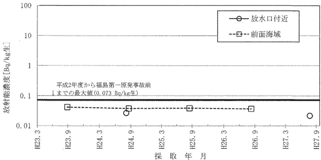
図-2-26 アラメのSr-90濃度の推移
