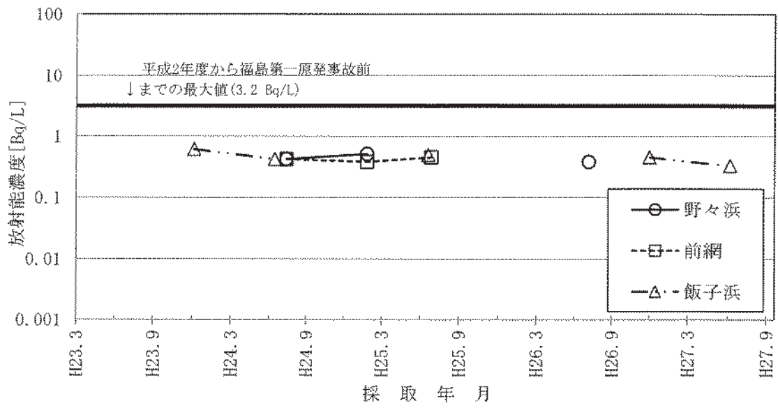
図-2-27 陸水のH-3濃度の推移
