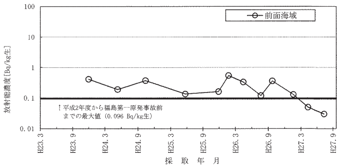
図-2-23 ムラサキガイのCs-137濃度の推移
