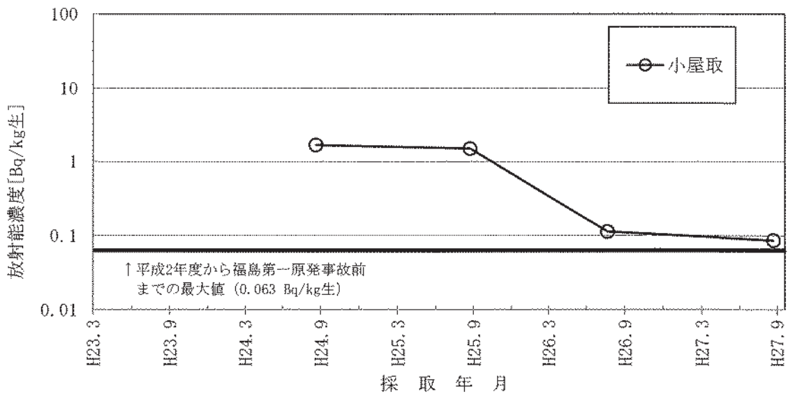
図-2-20 ウニのCs-137濃度の推移
