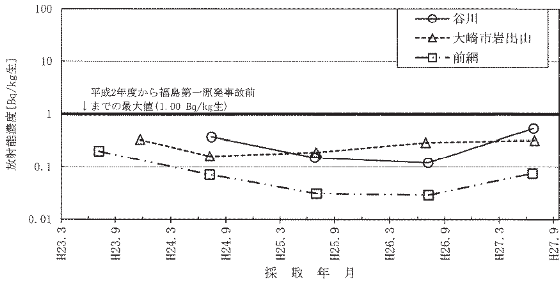
図-2-25 ヨモギのSr-90濃度の推移
