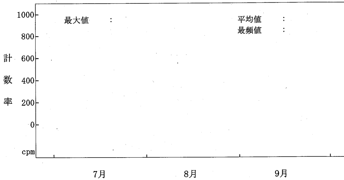
図-2-12 海水(放水)中の全ガンマ線計数率監視結果(1号機放水口モニター) (注) 7月1日~9月30日の欠測は、東日本大震災の影響によるもの。
