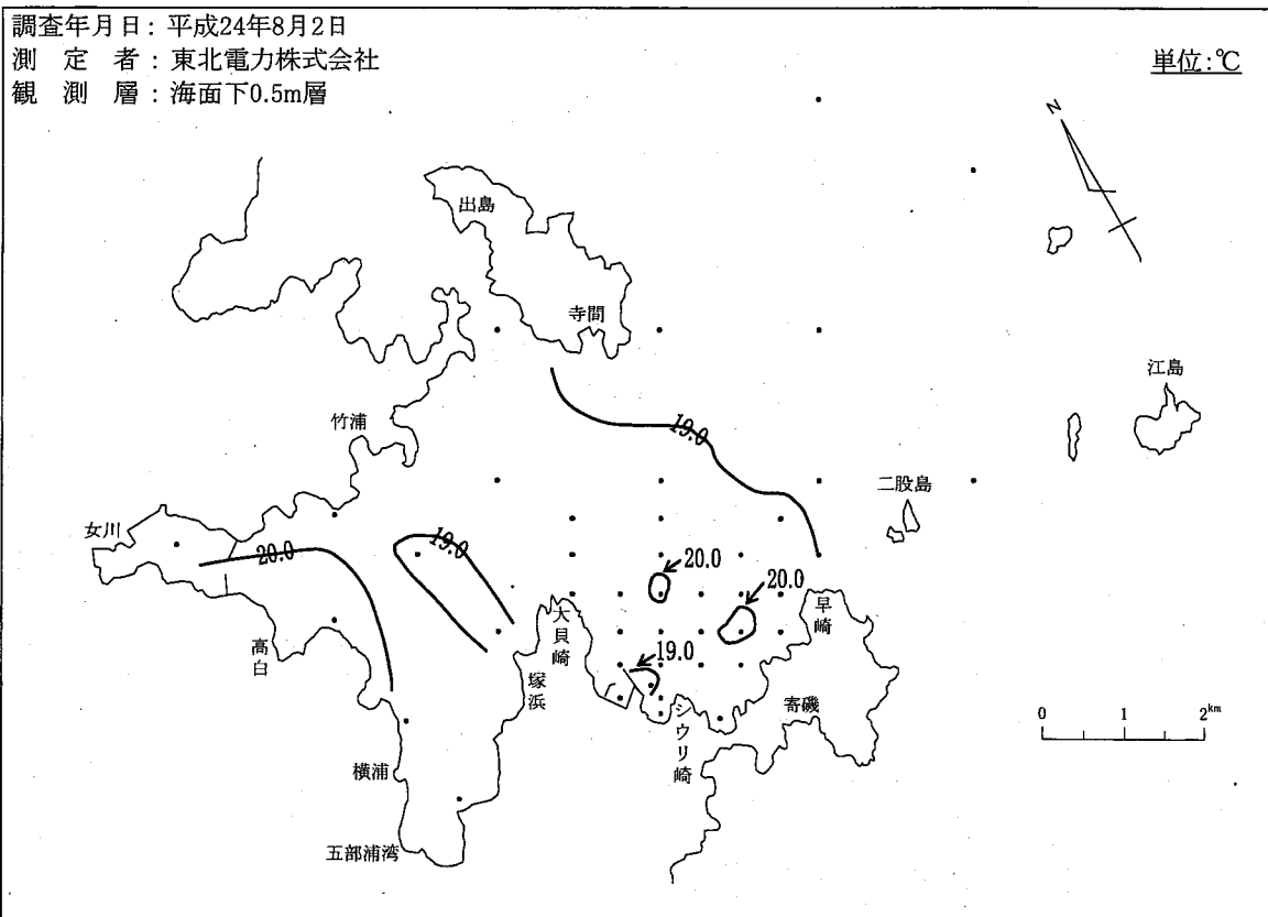
図-4-(2) 等温線
