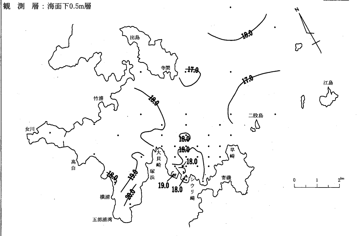
図-2-(2) 等温線
